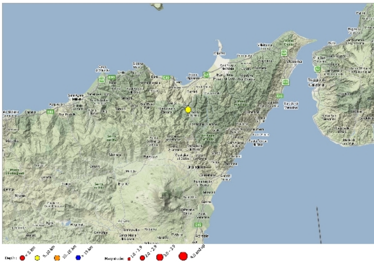
Fig. 1.2 Mappa della sismicità per la settimana 20-26 Dicembre relativa alle aree delle isole Eolie, Sicilia sudorientale, Sicilia nordorientale e Calabria meridionale.
