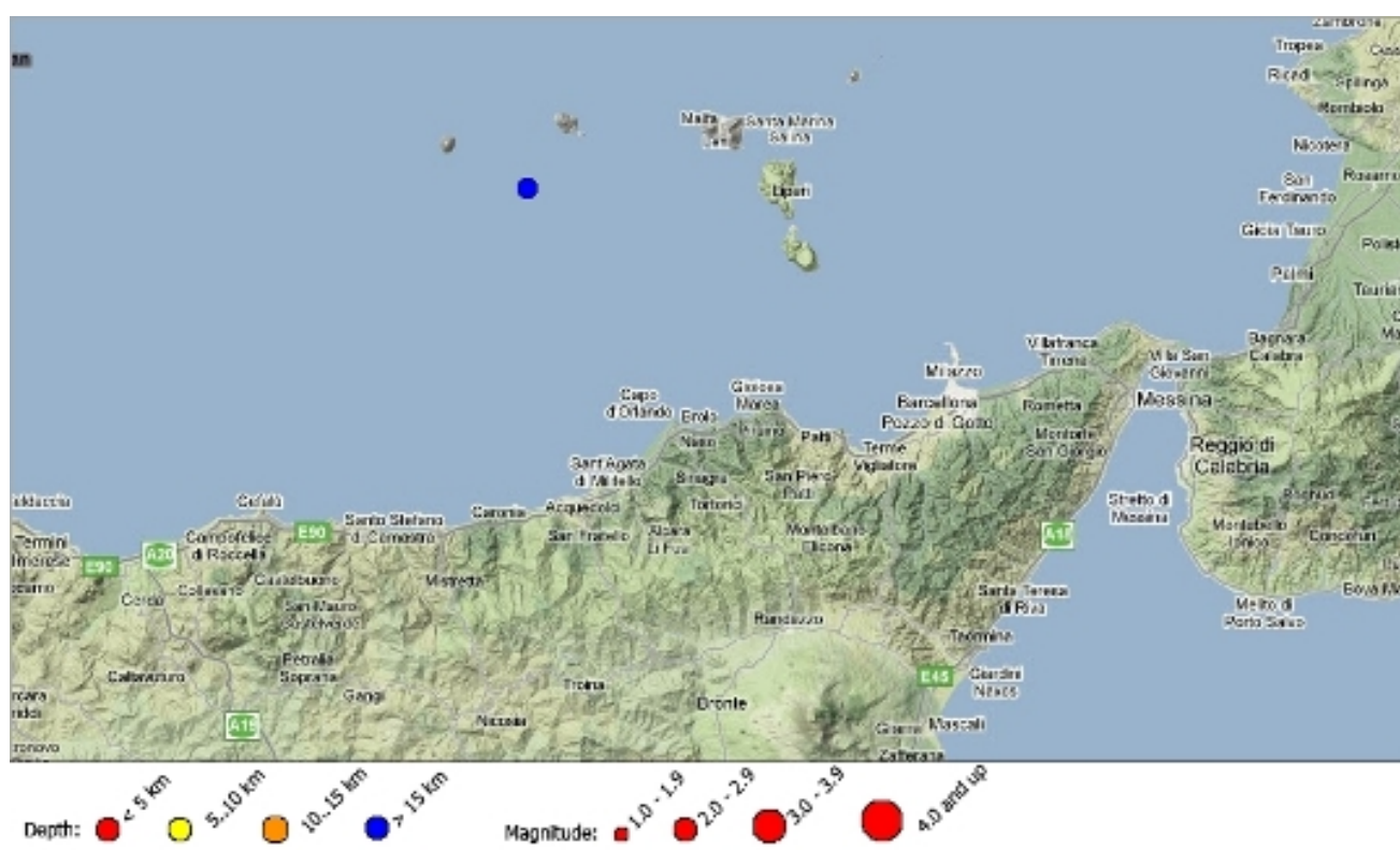
Fig. 1.2 Mappa della sismicità localizzata nell'area della Sicilia meridionale e nell'area della Sicilia Nord-Orientale e Calabria meridionale nella settimana 13 - 19 dicembre 2010.
