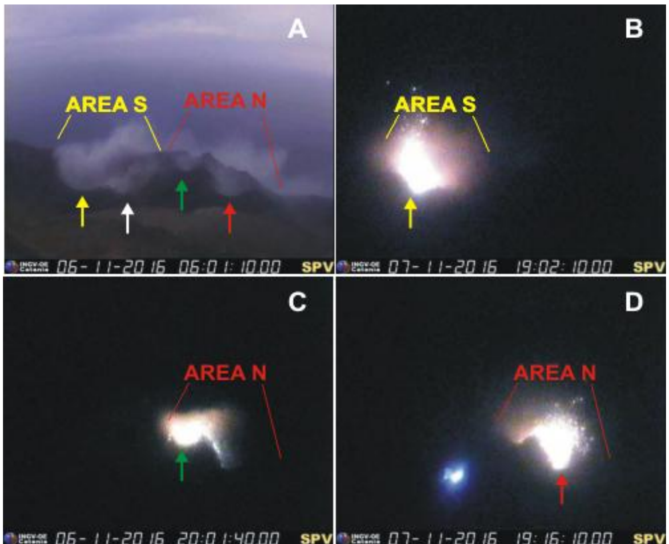
Fig. 1.1 A) Le principali bocche attive nella terrazza Craterica. Le frecce gialla e bianca indicano rispettivamente la bocca meridionale e settentrionale dell'area sud della Terrazza; le frecce verde e rossa indicano rispettivamente le bocche meridionale e settentrionale dell'area nord della Terrazza. B) esplosione con lancio di bombe dalla bocca meridionale (freccia gialla) dell'area sud della Terrazza Craterica. C) esplosione dalla bocca meridionale (freccia verde) dell'area nord della Terrazza. D) bocca settentrionale (freccia rossa) dell'area nord della Terrazza che produce un'esplosione con lancio di materiale balistico. Tutte le immagini sono riprese dalla telecamera visibile del Pizzo Sopra La Fossa.
