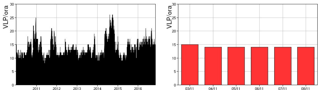
Fig. 4.3 Media giornaliera dell'ampiezza del tremore alla stazione STR9 dal 1/1/2010 (sinistra) e nell'ultima settimana (destra).
