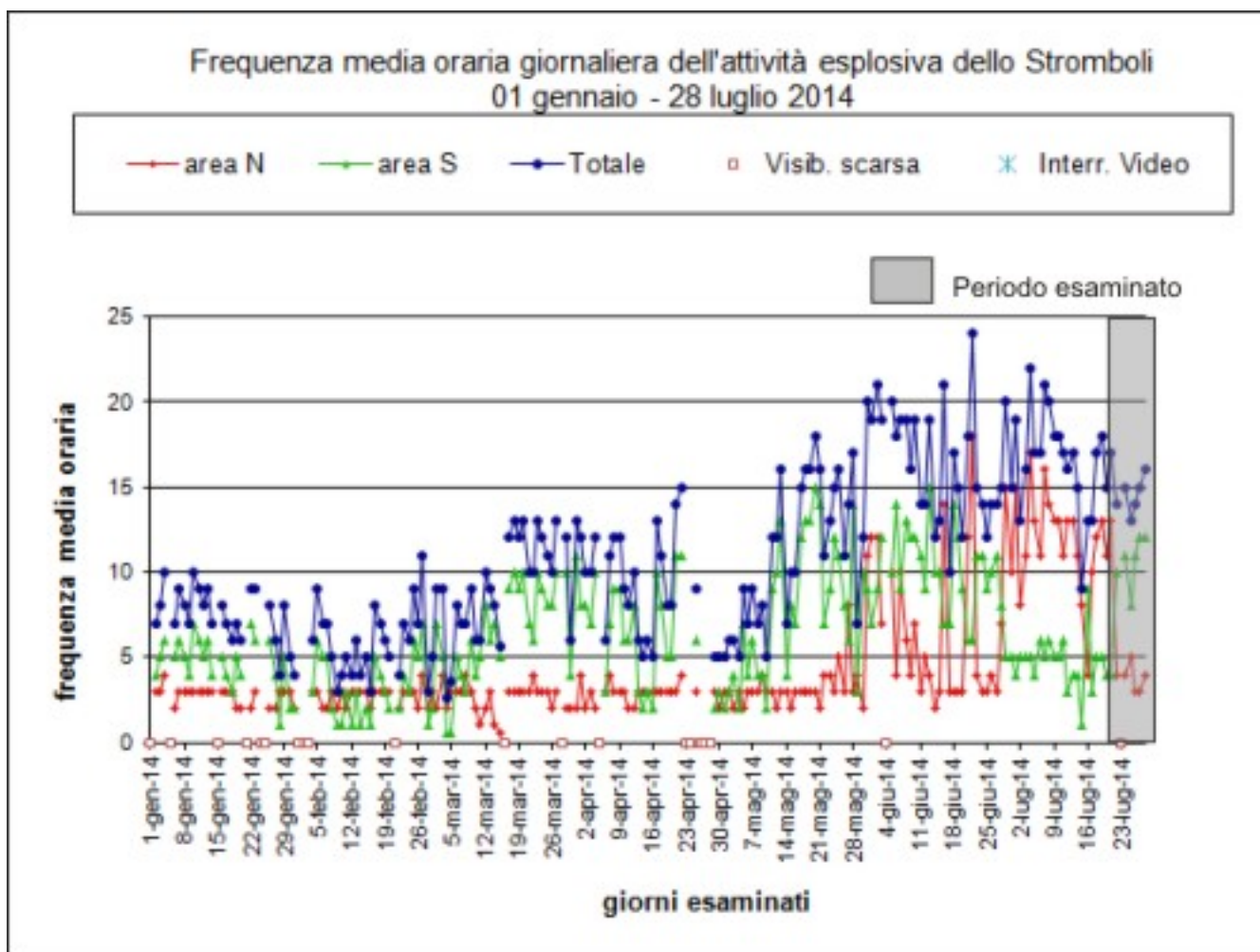
Fig. 1.2 Andamento della frequenza oraria media giornaliera degli eventi esplosivi dal 1 gennaio 2014, in grigio il periodo esaminato.
