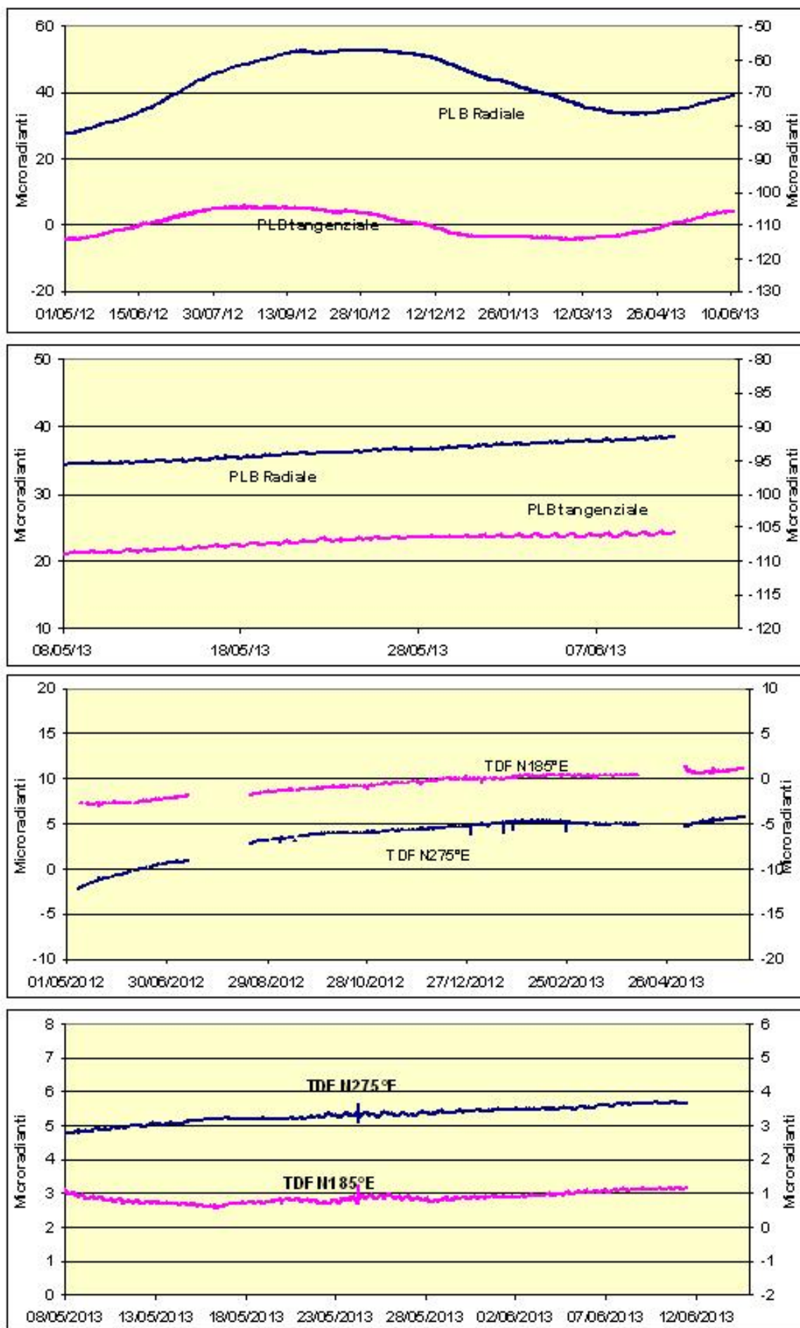
Fig. 3.1 Variazione dell'inclinazione del suolo alle stazioni clinometriche di PLB e TDF. In alto la componente radiale e tangenziale di PLB nel lungo e nel breve periodo. Analogamente in basso
