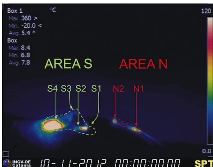
Fig. 1.1 La terrazza craterica vista dalla telecamera termica posta sul Pizzo sopra la Fossa. Le
