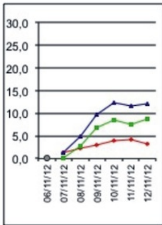
Fig. 1.2 Andamento della frequenza oraria media giornaliera degli eventi esplosivi nel periodo osservato (ingrandito in basso).
