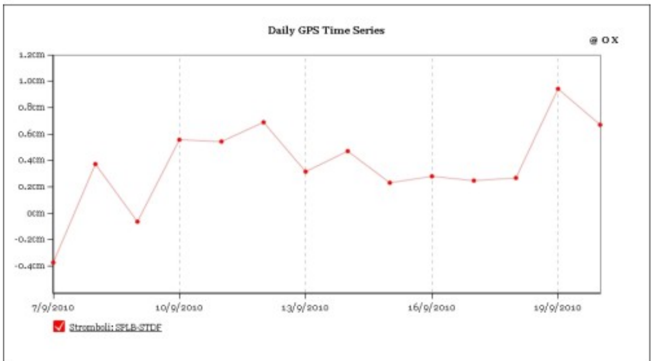
Fig. 3.2 Variazione della Distanza Reale (Slope Distance) tra le stazioni GPS permanenti di Punta Labronzo (SPLB) e Timpone del Fuoco (STDF), nei due intervalli di un anno (in alto) e di due settimane (in basso).
