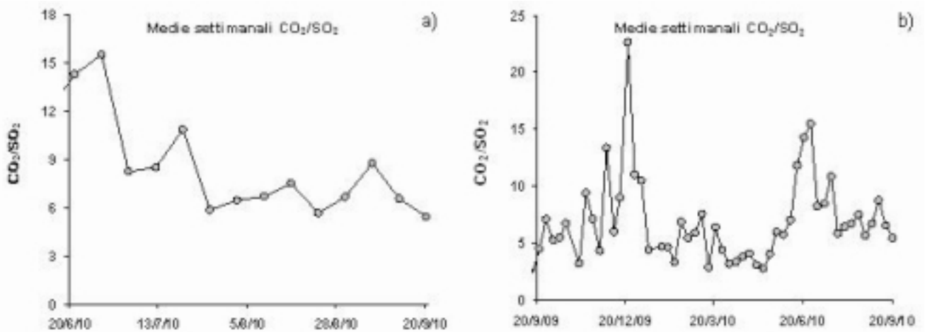
Fig. 2.2 Andamento temporale del rapporto CO 2 /SO 2 nel plume: ultimi tre mesi (a), ultimo anno (b).
