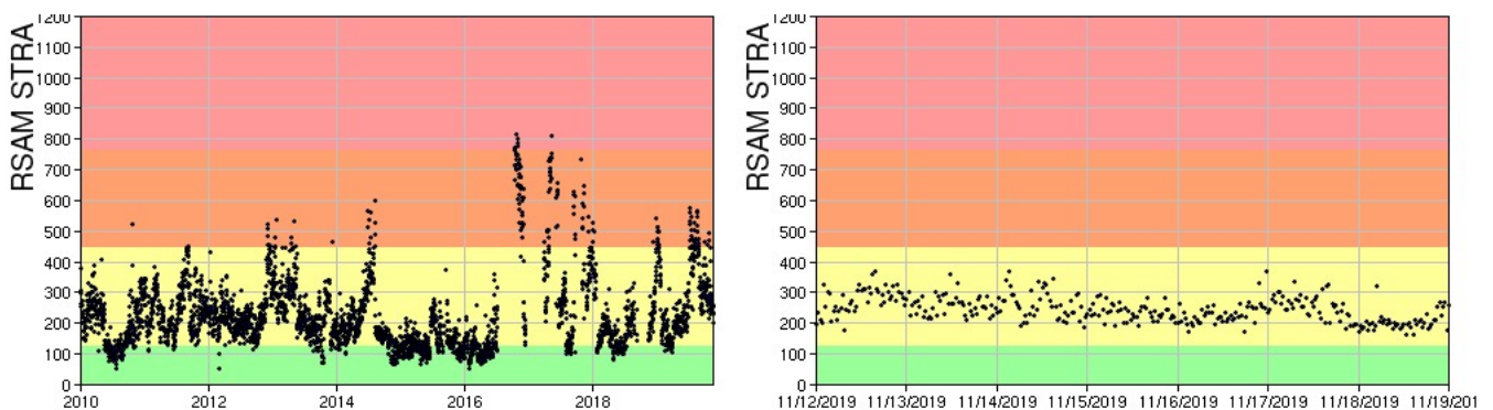
Fig. 4.2 - Media giornaliera dell'ampiezza del tremore alla stazione STR1 dal 1/1/2010 (sinistra) e nell'ultima settimana (destra).
