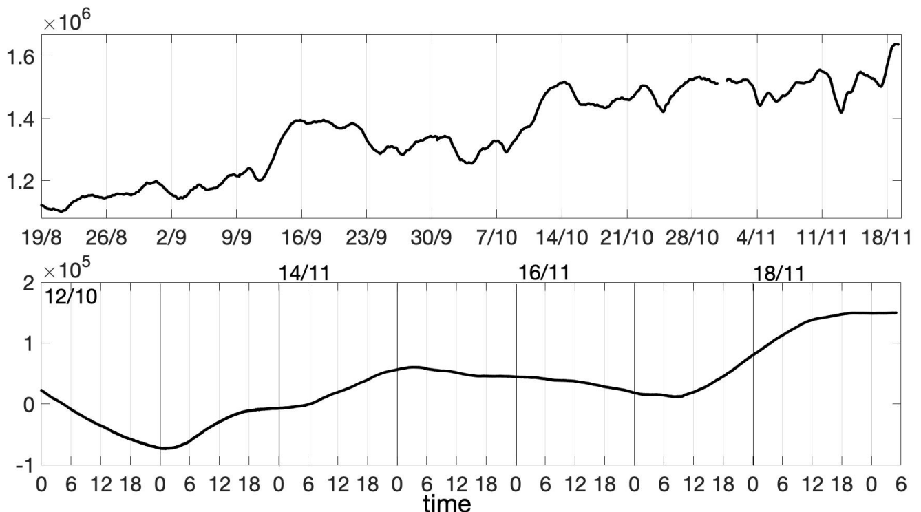
Fig. 4.4 - Grafico relativo al dato dilatometrico registrato a SVO: in alto viene mostrato lo strain registrato dal 19/08 2019, in basso quello nell'ultima settimana.
