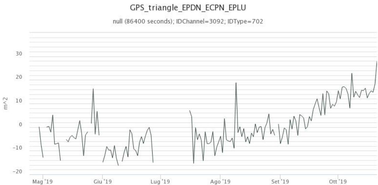
Fig. 6.1 - Serie temporale della variazione di dilatazione areale del triangolo sommitale EPDN-ECPN-EPLU
