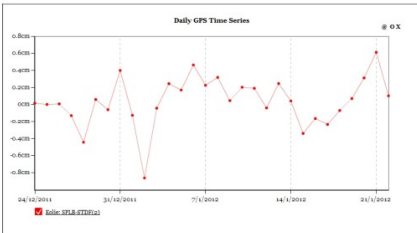
Fig. 3.1 Variazione della Distanza Reale (Slope Distance) tra le stazioni GPS permanenti di Punta Labronzo (SPLB) e Timpone del Fuoco (STDF), nei due intervalli di un anno (in alto) e di un mese (in basso).
