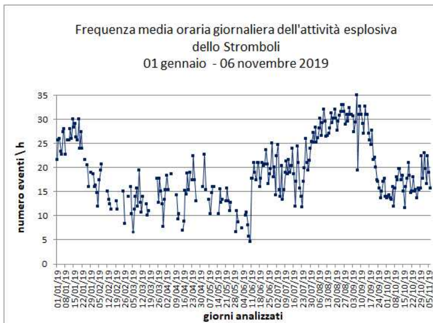
Fig. 3.1 - Frequenza media oraria giornaliera totale delle esplosioni dello Stromboli tra gennaio e novembre 2019 (dato aggiornato al 6 novembre)
