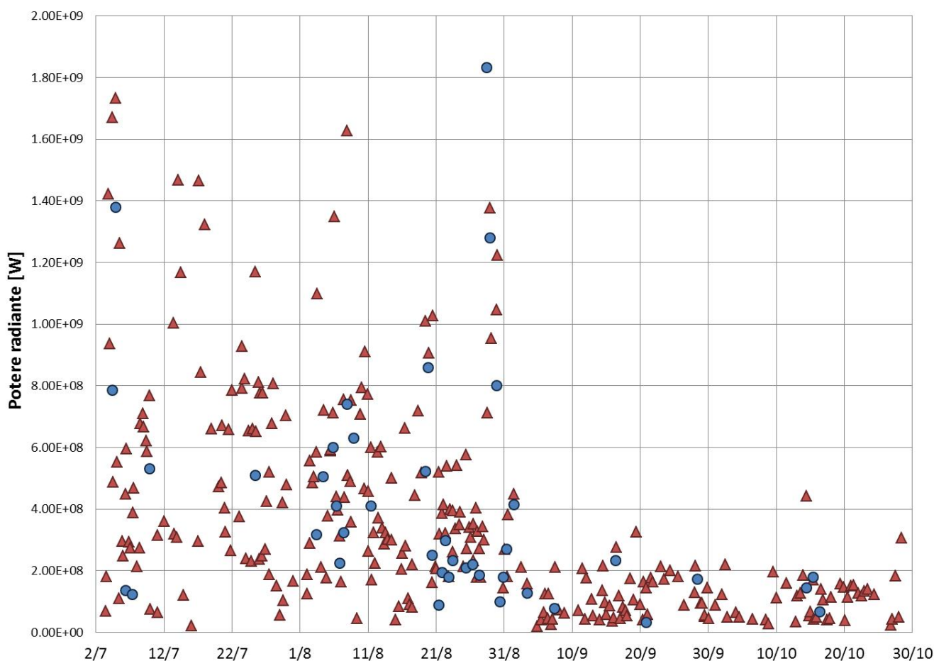
Fig. 7.1 - Fig. 7.1 –Flusso radiante calcolato da dati MODIS (triangolo rosso) e Sentinel-3 SLSTR (cerchio blu) dal 3 luglio al 28 ottobre.
