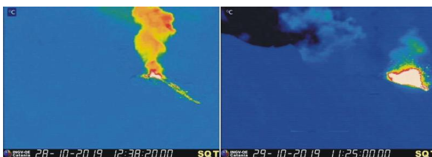
Fig. 3.1 - A sinistra: immagine termica di un'esplosione da una delle bocche presenti nell'area Nord della terrazza craterica, con rotolamento del materiale grossolano lungo i fianchi del cono prospiciente la Sciara del Fuoco. A destra: immagine termica di un'esplosione da una delle bocche presenti nell'area Centro-Sud della terrazza craterica. Immagini registrate dalle telecamere di sorveglianza di quota 400 m sul lato nord della Sciara del Fuoco.
