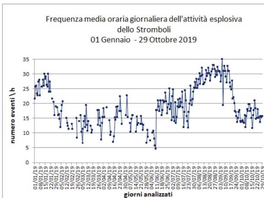
Fig. 3.2 - Frequenza media oraria giornaliera totale delle esplosioni dello Stromboli durante l'anno 2019 (conteggio aggiornato al 29 ottobre).
