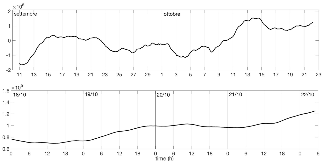
Fig. 4.3 - Grafico relativo al dato dilatometrico registrato alla stazione SVO: in alto viene mostrato lo strain registrato dal 11/09/2019, in basso quello relativo al periodo dal 18/10 al 22/10.
