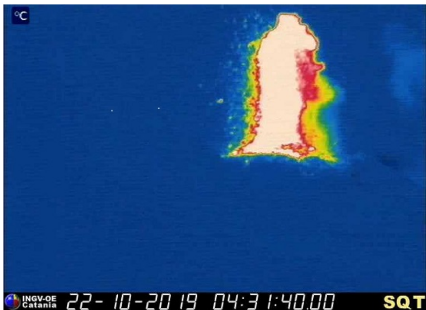
Fig. 3.2 - Immagine termica di un'esplosione dell'area N, le riprese sono da quota 400 m (s.l.m).
