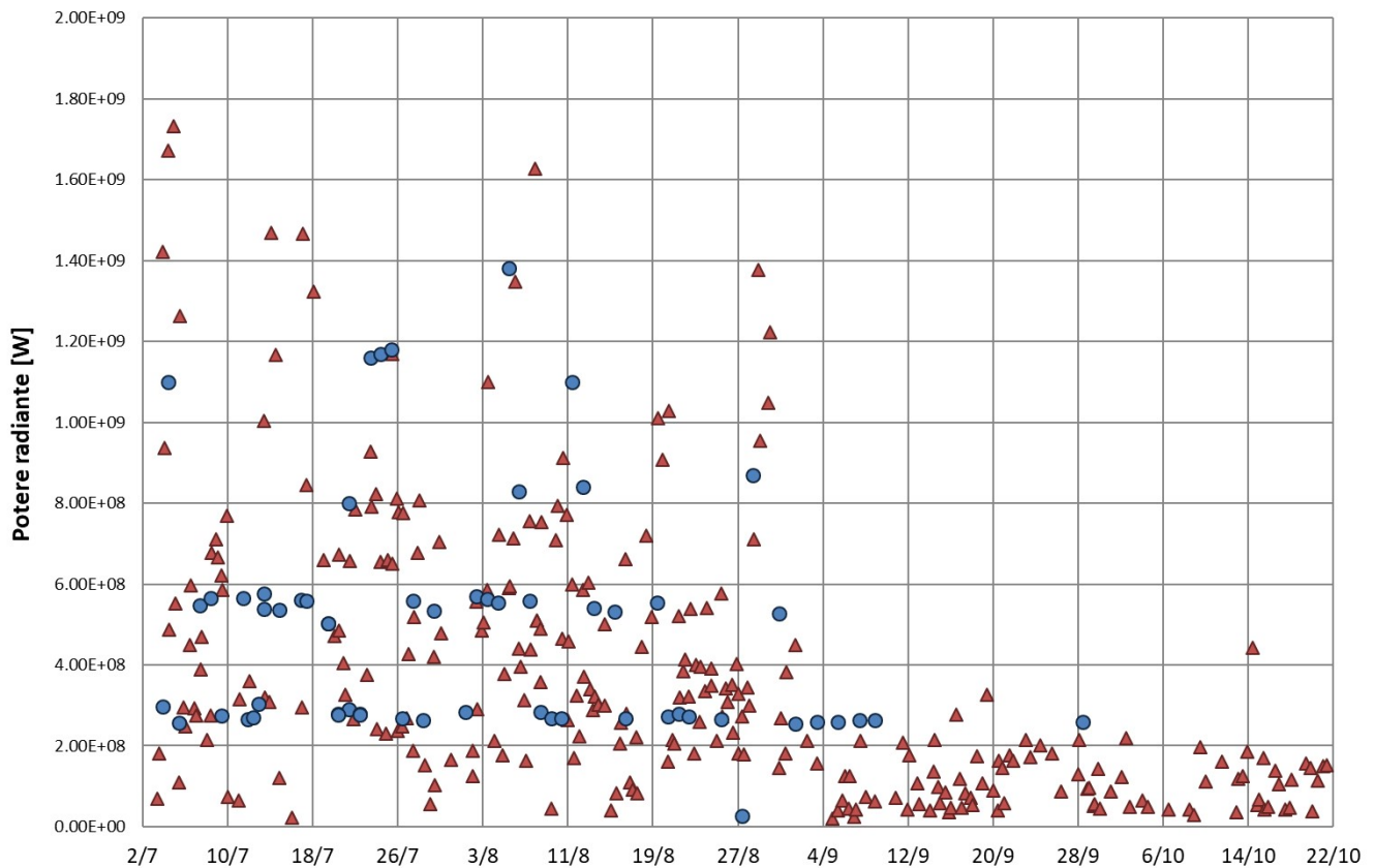
Fig. 7.1 - Flusso radiante calcolato da dati MODIS (triangolo rosso) e Sentinel-3 SLSTR (cerchio blu) dal 3 luglio al 21 ottobre.
