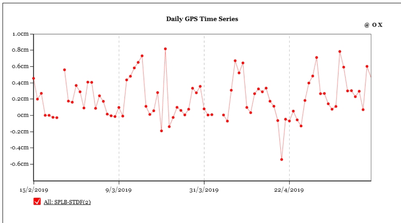
Fig. 5.1 - Serie temporale della variazione di distanza tra le stazioni STDF e SPLB
