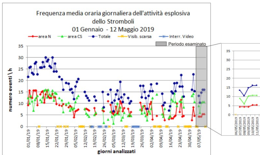
Fig. 3.2 - Grafico della frequenza oraria media giornaliera degli eventi esplosivi ripresi dalle telecamere di sorveglianza dal 1 gennaio 2019. Il valore totale è la somma della frequenza oraria media giornaliera di tutti gli eventi esplosivi prodotti dalle bocche attive.
