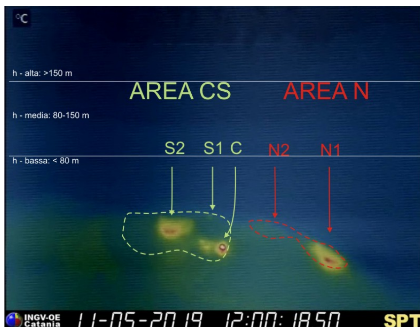
Fig. 3.1 - La terrazza craterica vista dalla telecamera termica posta sul Pizzo sopra la Fossa, le aree con i bordi tratteggiati indicano i settori della terrazza da cui si osserva l'attività esplosiva (AREA N, AREA C-S). Le sigle e le frecce indicano i nomi e le ubicazioni delle bocche attive. L'areale soprastante la terrazza craterica è diviso in tre intervalli di altezze ( h ) che indicano l'intensità dell'esplosioni.
