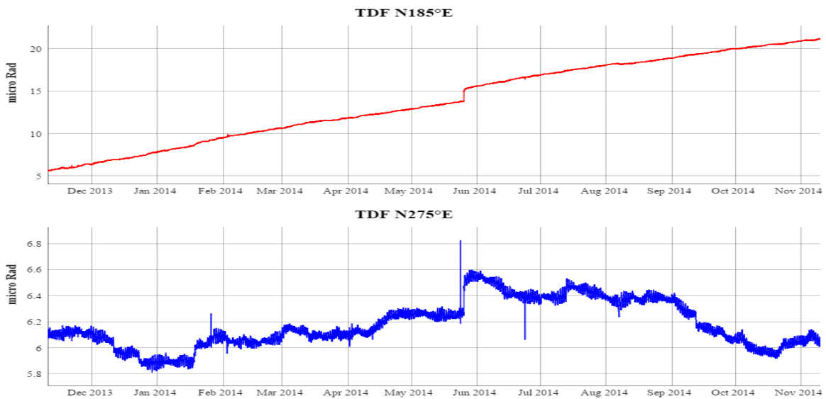
Figura 7– Dato clinometrico nel periodo compreso tra ottobre 2013 e novembre 2014.
