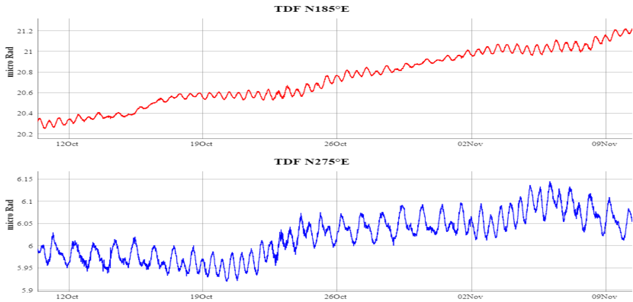
Figura 8– Dato clinometrico nel periodo compreso tra il 6 ottobre ed il 9 novembre 2014.
