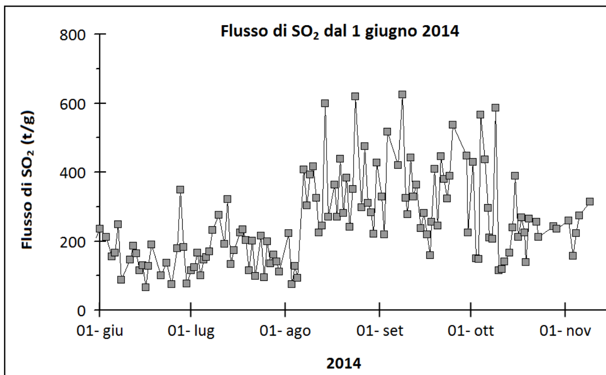
Figura 6 – Flusso di \text{SO}_2 medio-giornaliero dal 1 giugno 2014.
