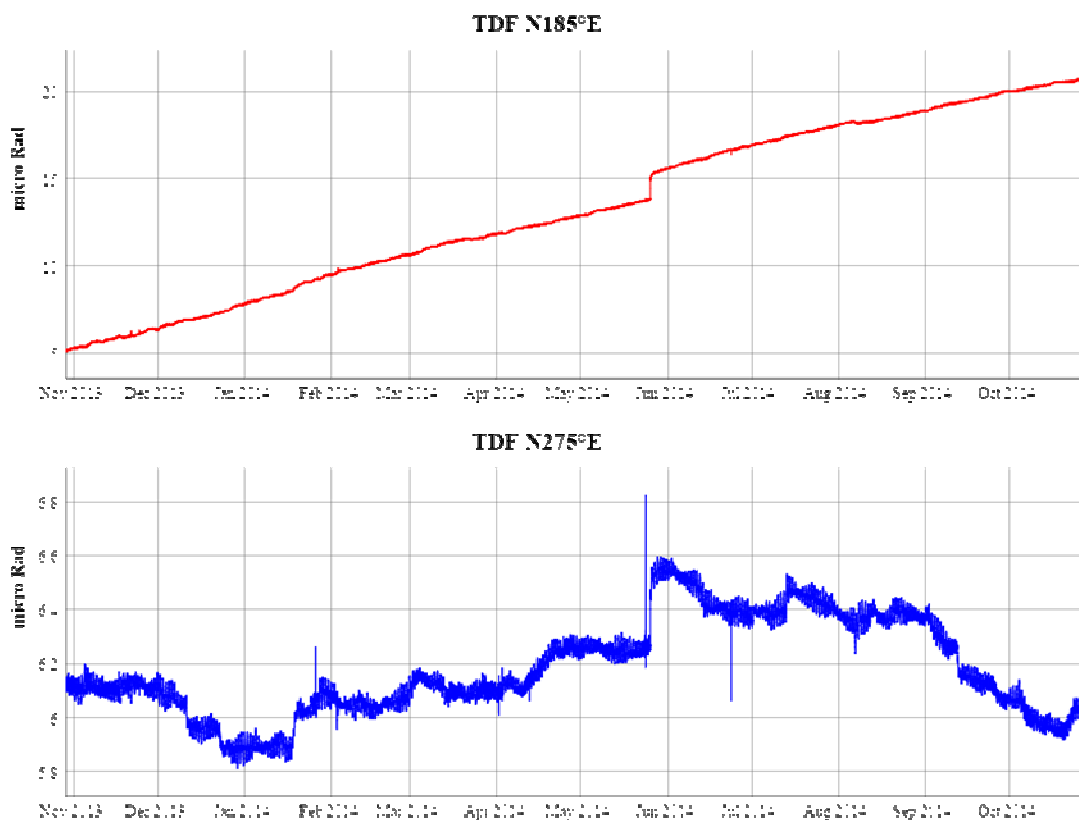
Figura 8 - Dato clinometrico nel periodo compreso tra ottobre 2013 ed il 27 ottobre 2014.
