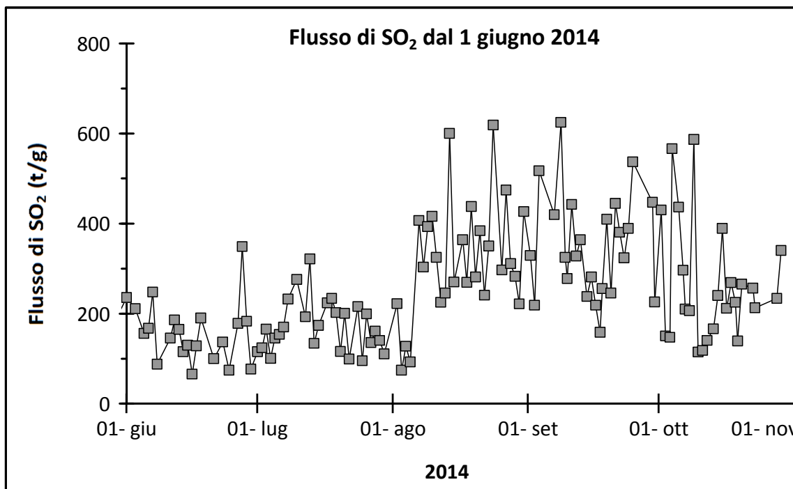
Figura 7 – Flusso di SO 2 medio-giornaliero dal 1 giugno del 2014.
