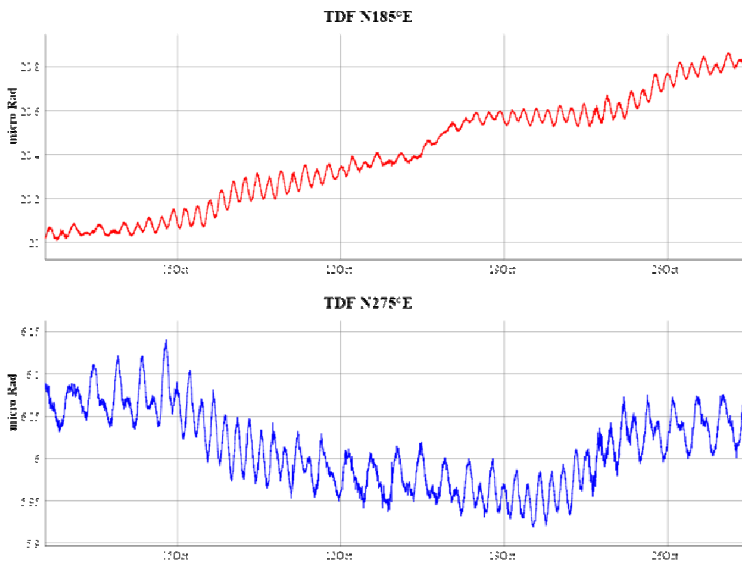
Figura 9 - Dato clinometrico nel periodo compreso tra il 14 settembre ed il 27 ottobre 2014.
