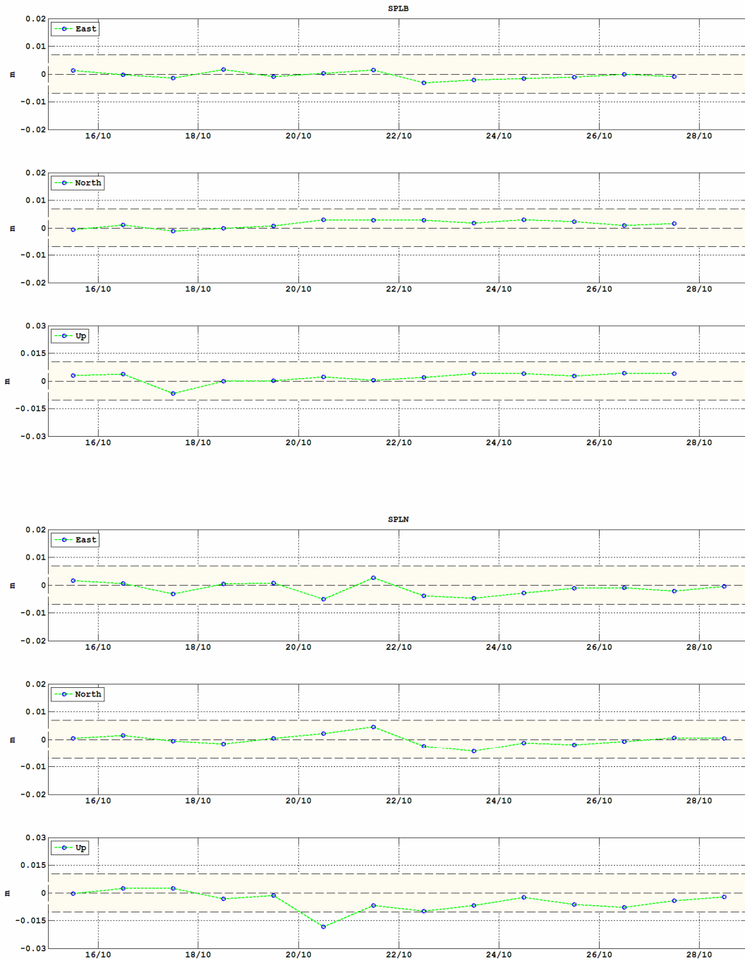
Figura 10 - Serie temporali delle componenti E-W, N-S e quota per gli ultimi 15 giorni delle stazioni CGPS dello Stromboli, calcolate attraverso il software RTD.
