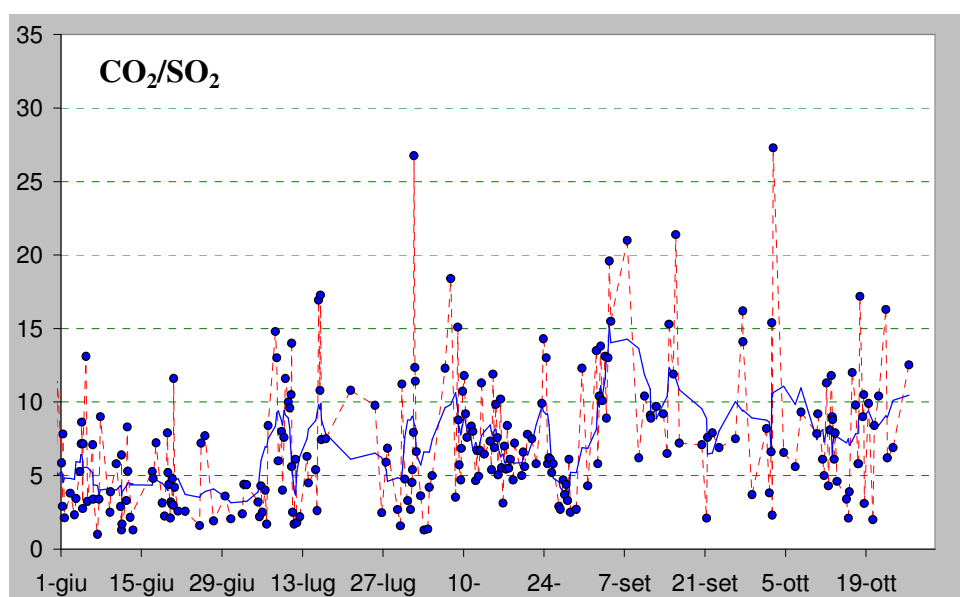
Figura 6– Rapporto CO 2 /SO 2 misurato nel plume vulcanico dello Stromboli nel periodo tra il 1 giugno ed il 26 ottobre 2014 (ultimo dato ore 13:30 locali del 26 ottobre).
