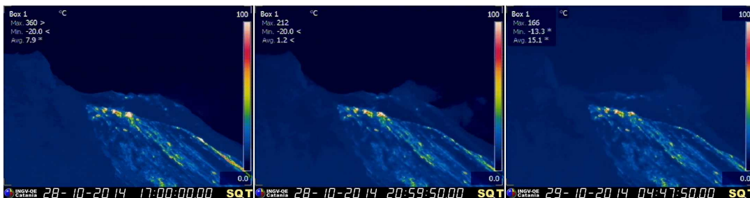
Figura 2 – Immagini visibili (in alto) e termiche (in basso) riprese dalle telecamere di quota 400 m s.l.m. che mostrano le fasi di raffreddamento del campo lavico nella giornata del 28 e 29.
