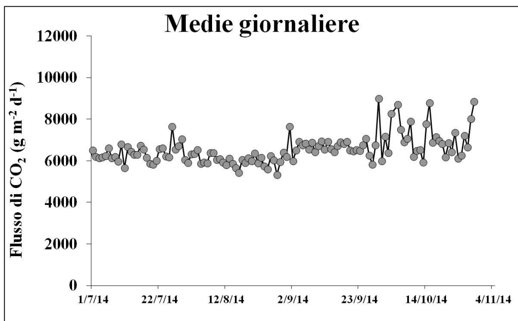
Figura 5 – Flusso medio-giornaliero di CO 2 dal suolo dal 01 luglio al 29 ottobre 2014.
