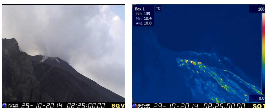
Figura 3 – Immagini visibili e termiche riprese dalle telecamere di quota 400 m s.l.m. che mostrano le anomalie nella parte alta della Sciara del Fuoco.
