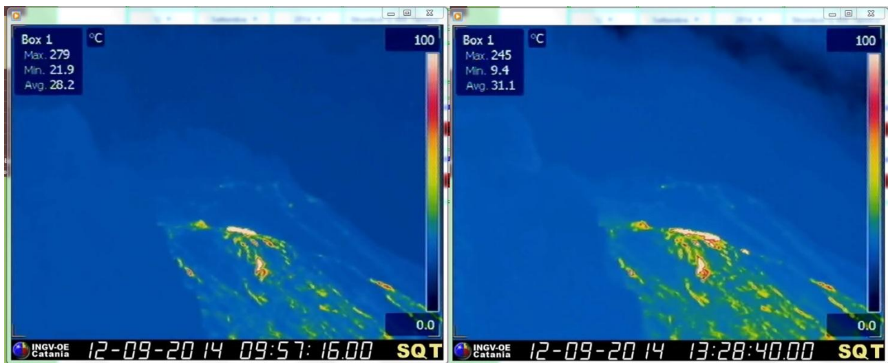
Figura 1 Le immagini della telecamera termica di quota 400 m mostrano il campo lavico che si riversa a 600 m di quota.
