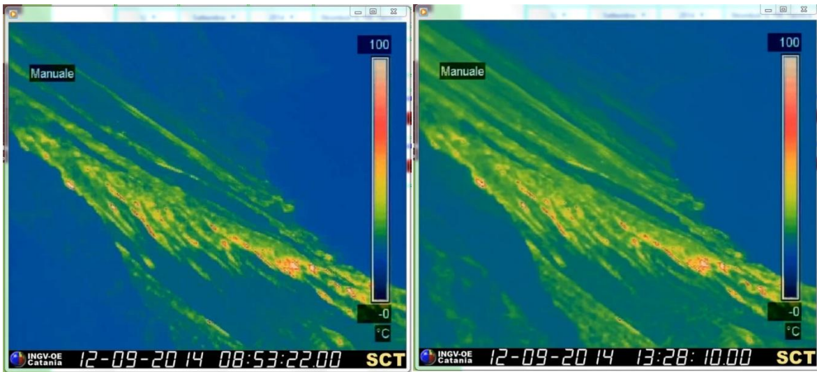
Figura 2 Nelle immagini termiche della telecamera di quota 190 m è visibile la parte più bassa del campo lavico in raffreddamento che non presenta variazioni di rilievo rispetto a stamattina.
