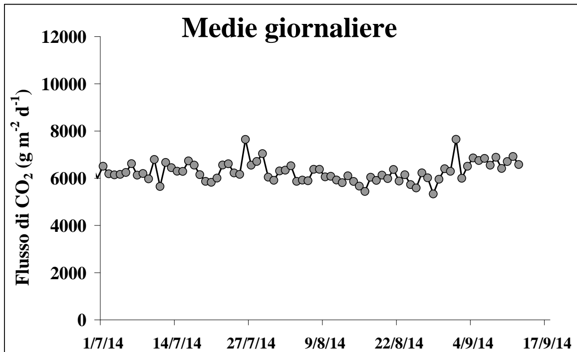
Figura 3 – Flusso medio-giornaliero di CO 2 dal suolo nel periodo tra il 1 luglio ed il 12 settembre 2014
