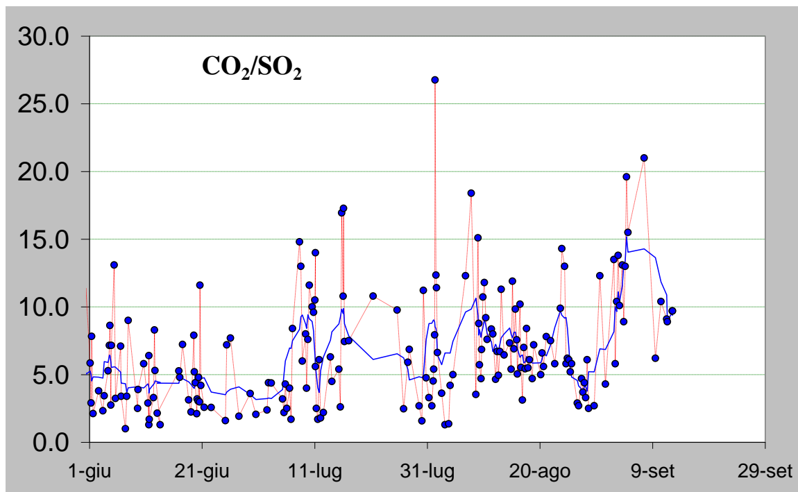
Figura 4 – Rapporto \text{CO}_2/\text{SO}_2 misurato nel plume vulcanico dello Stromboli nel periodo tra il 1 giugno ed il 12 settembre 2014 (ultimo dato ore 15:30 locali del 12 settembre).
