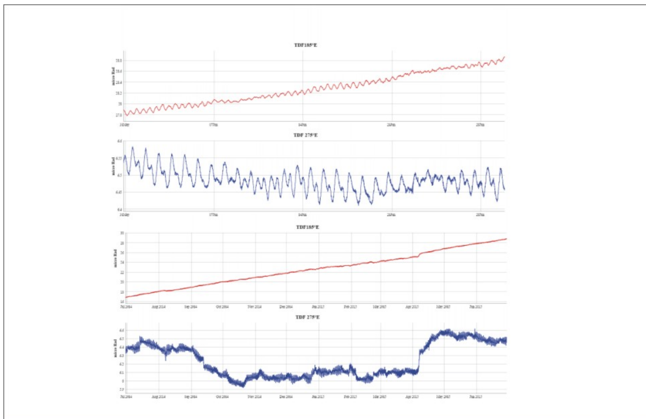
Fig. 3.1 Variazione dell'inclinazione del suolo alla stazione clinometrica di TDF. Sono riportate le componenti N185°E (in rosso) e N275° (in blu) di TDF nel breve (un mese, in alto) e nel lungo periodo (un anno, in basso).
