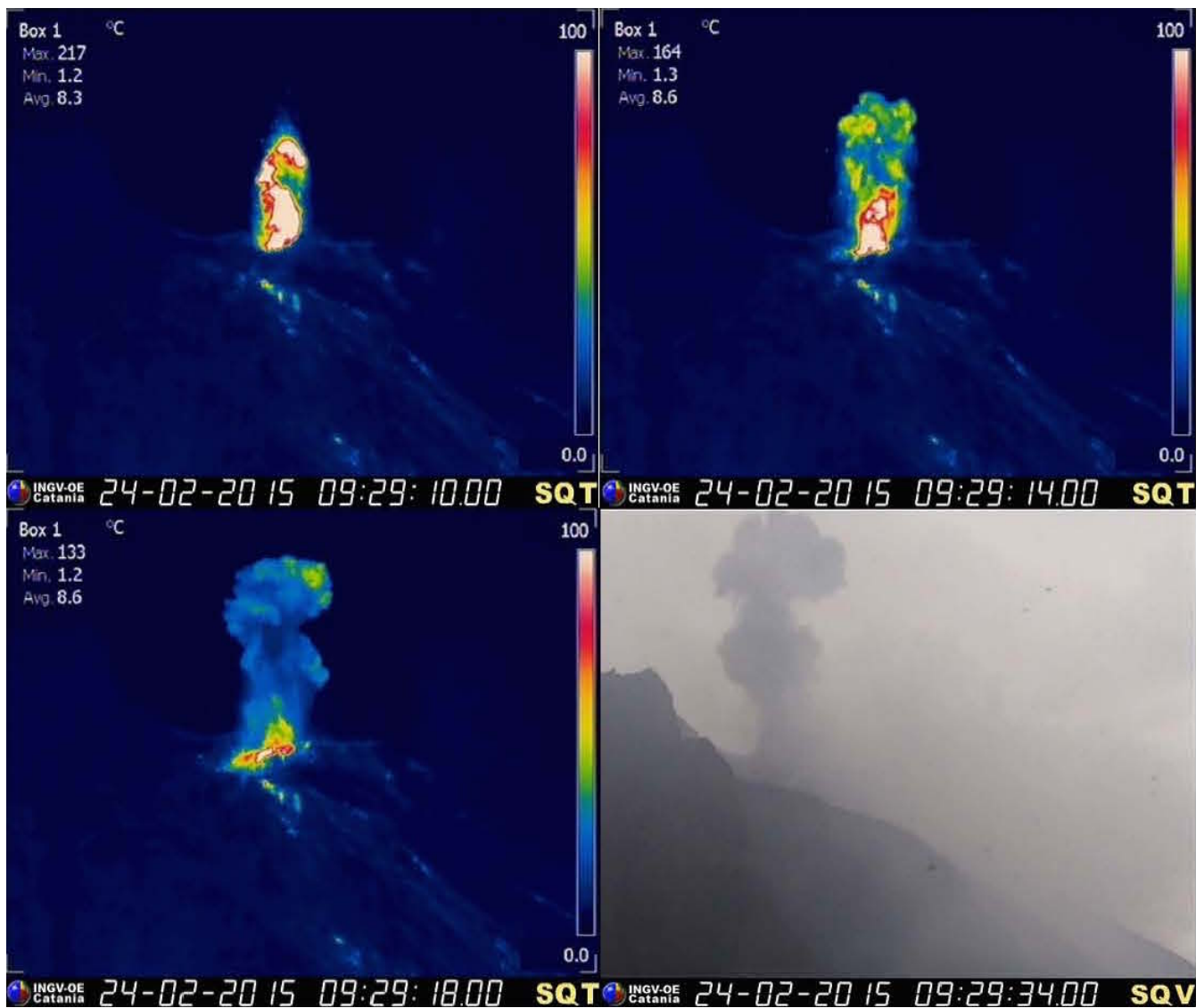
Fig. 1.1 Immagini termiche dell'esplosione stromboliana più intensa rilevata in questo periodo, prodotta il 24 febbraio dalla bocca più settentrionale della Terrazza Craterica.
