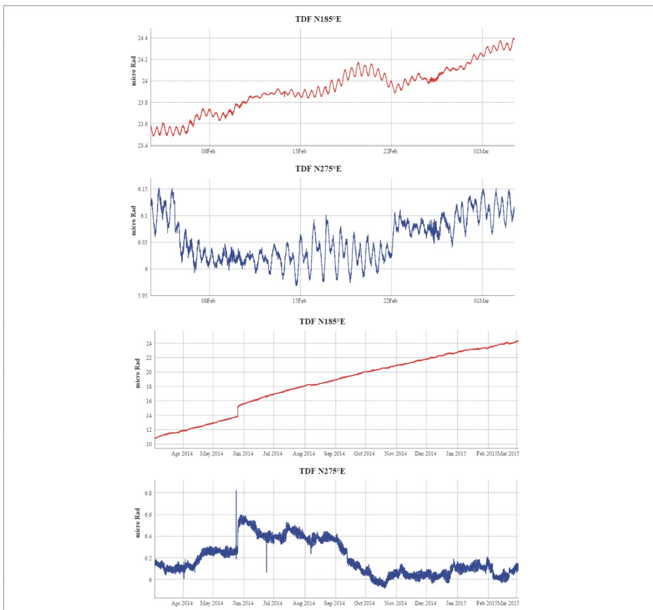
Fig. 3.1 Variazione dell'inclinazione del suolo alla stazione clinometrica di TDF. Sono riportate le componenti N185°E e N275°le di TDF nel breve (un mese) e nel lungo (un anno) periodo.
