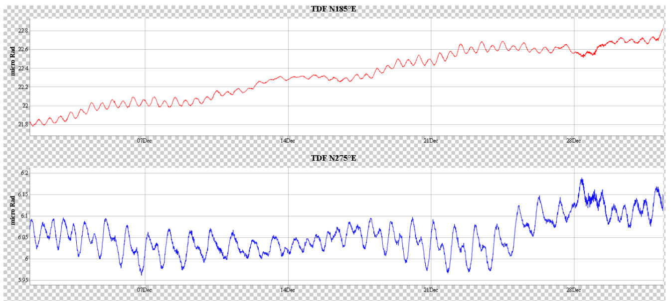
Fig.9 – Dato clinometric nel periodo compreso tra il 30 novembre 2014 e il 01 gennaio 2015
