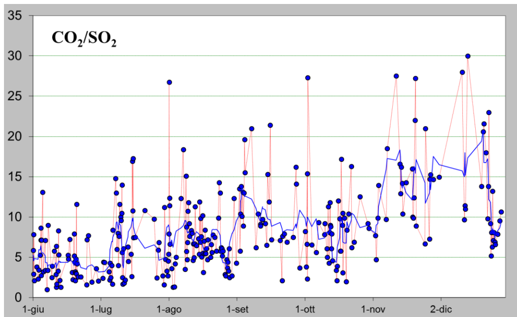
Figura 3– Rapporto CO 2 /SO 2 misurato nel plume vulcanico dello Stromboli nel periodo tra il 1 giugno e il 28 dicembre 2014 (ultimo dato ore 23:30 GMT del 28 dicembre).
