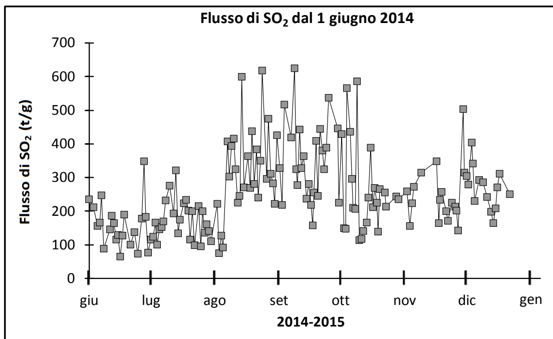
Figura 4 – Flusso di SO 2 medio-giornaliero dal 1 giugno 2014.
