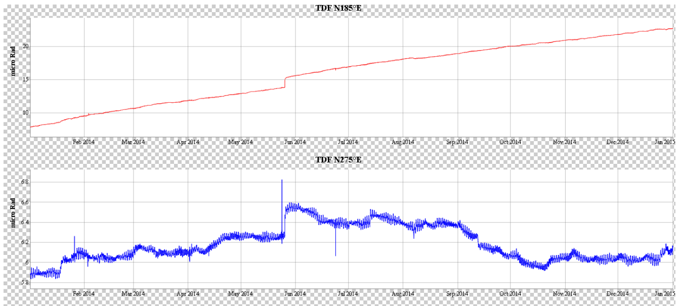
Fig.8– Dato clinometric nel periodo compreso tra gennaio 2014 e gennaio 2015
