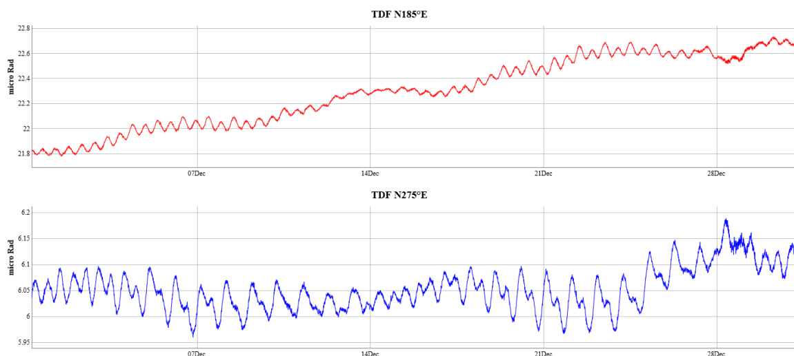
Fig.9 – Dato clinometrico nel periodo compreso tra il 30 novembre e il 29 dicembre 2014
