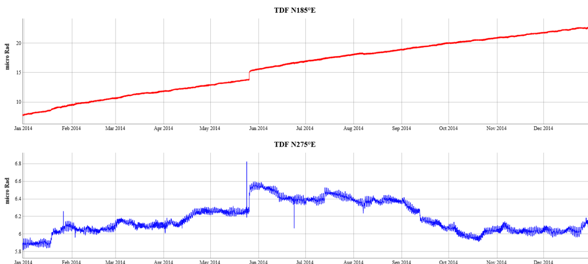
Fig.8– Dato clinometrico nel periodo compreso tra gennaio e dicembre 2014
