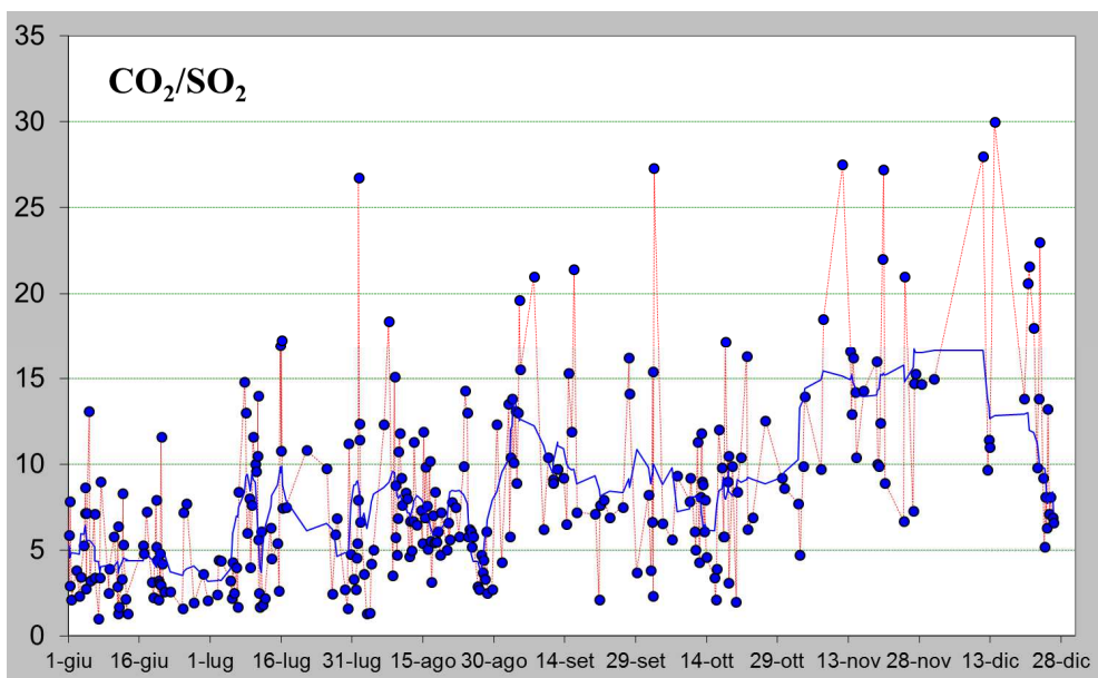
Figura 3 – Rapporto CO 2 /SO 2 misurato nel plume vulcanico dello Stromboli nel periodo tra il 1 giugno e il 26 dicembre 2014 (ultimo dato ore 12:30 locali del 26 dicembre).
