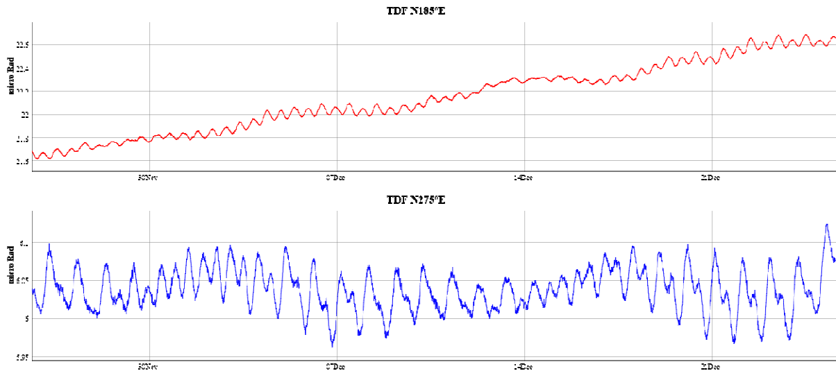
Figura 10 – Dato clinometrico nel periodo compreso tra novembre e dicembre 2014.
