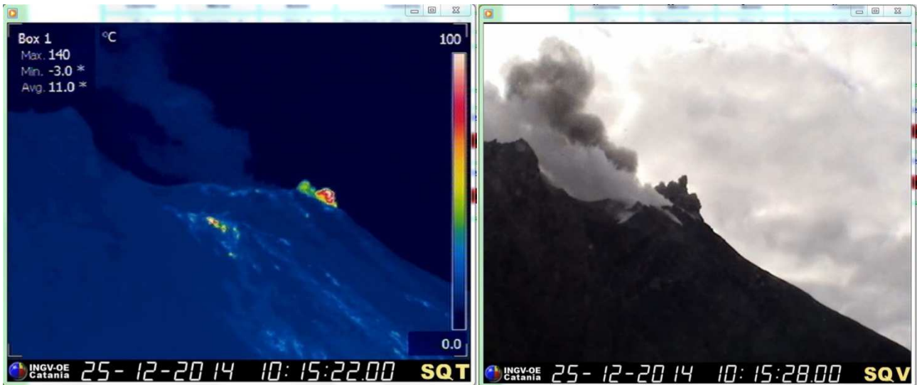
Figura 2 – Immagini riprese dalla telecamera termica e visibile di quota 400 m s.l.m. degli eventi esplosivi con emissione di cenere.
