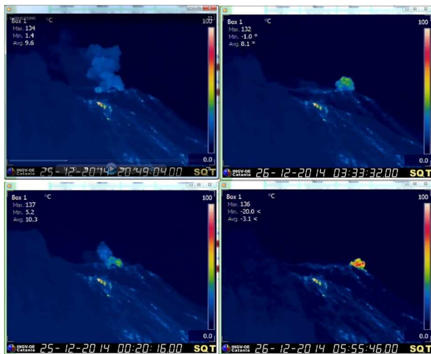
Figura 1 – Immagini riprese dalla telecamera termica di quota 400 m s.l.m. degli eventi esplosivi osservati.
