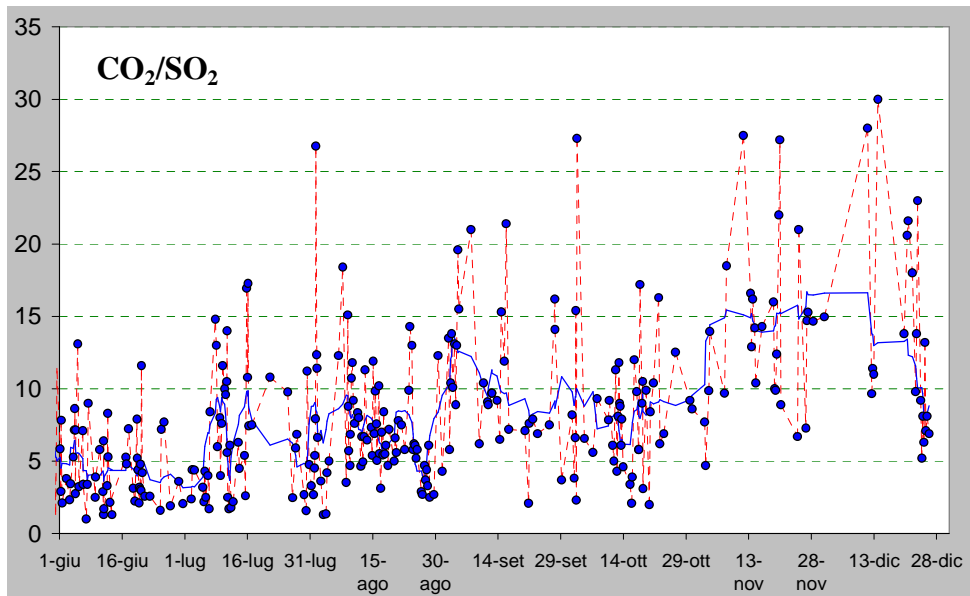
Figura 4– Rapporto CO_2/SO_2 misurato nel plume vulcanico dello Stromboli nel periodo tra il 1 giugno e il 26 dicembre 2014 (ultimo dato ore 6:30 locali del 26 dicembre).
