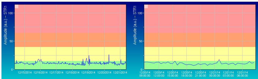
Ampezza del tremore alla stazione STR1 nell'ultima settimana (sinistra) e nelle ultime 24h (destra)
