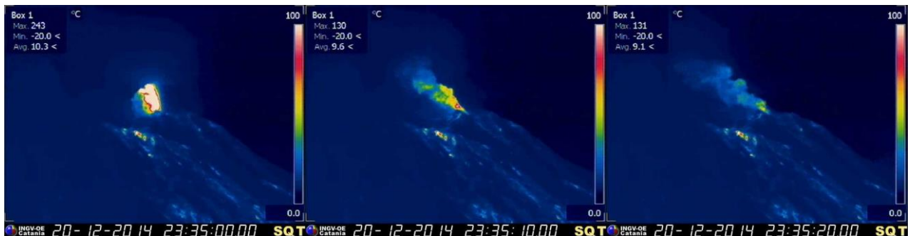
Figura 1 – Immagini riprese dalla telecamera termica di quota 400 m s.l.m. che mostrano l'evento esplosivo più forte registrato il 20 dicembre durante la fase di bassa attività iniziata dopo le 5 UTC.
