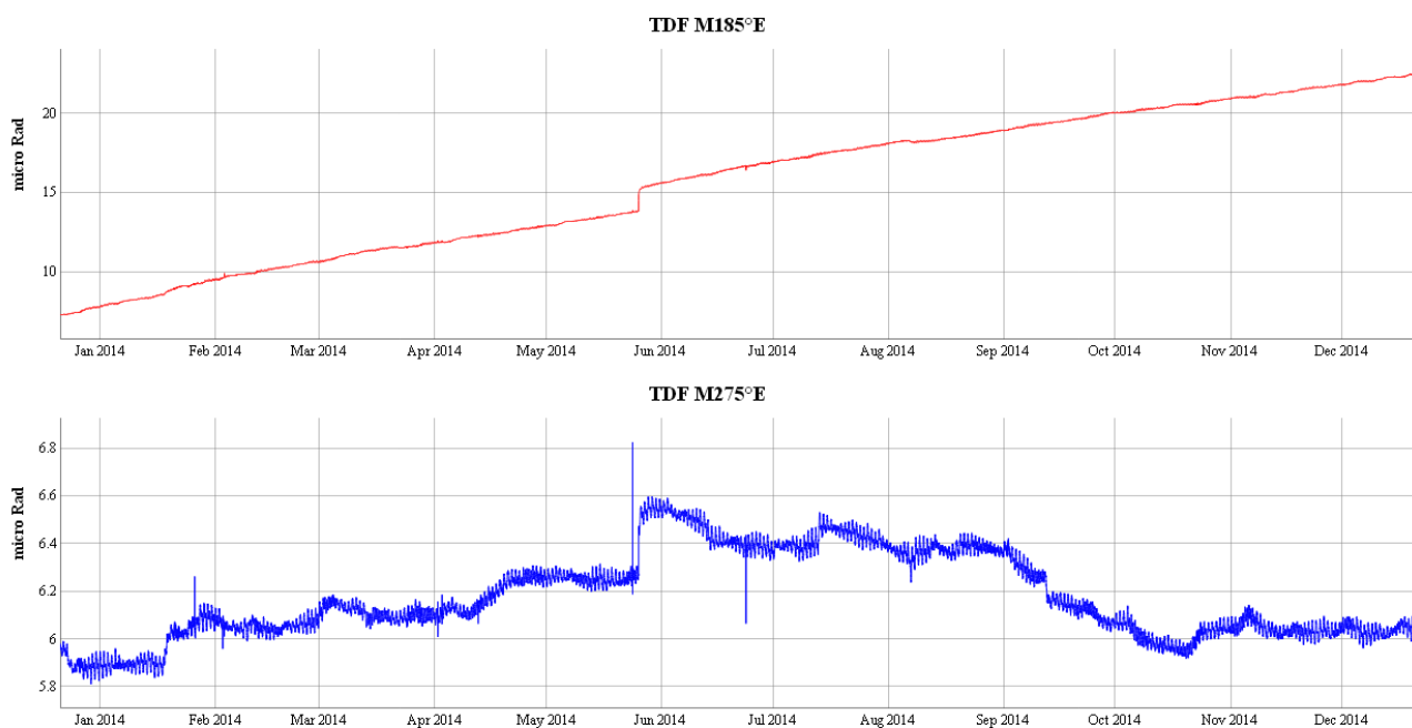
Figura 5 – Dato clinometrico nel periodo compreso tra dicembre 2013 e dicembre 2014.
