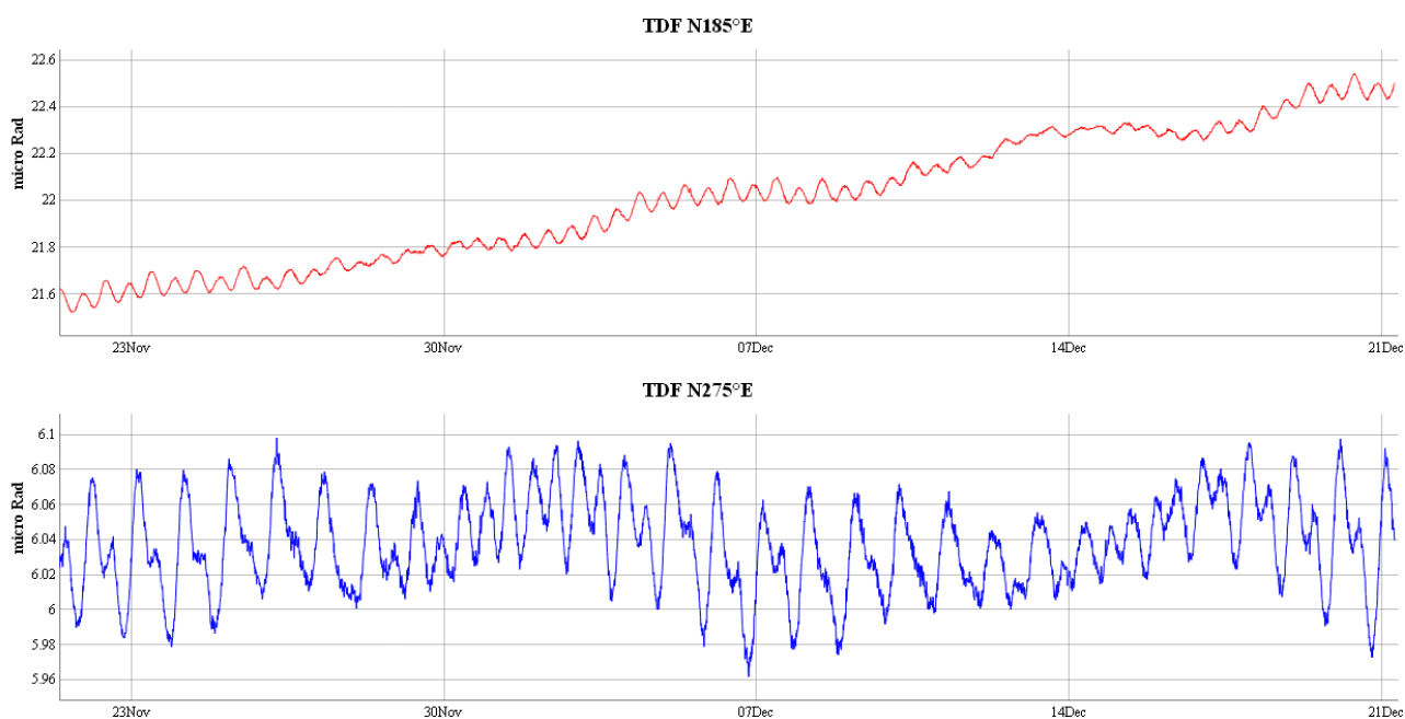
Figura 6 – Dato clinometrico nel periodo compreso tra novembre e dicembre 2014.
