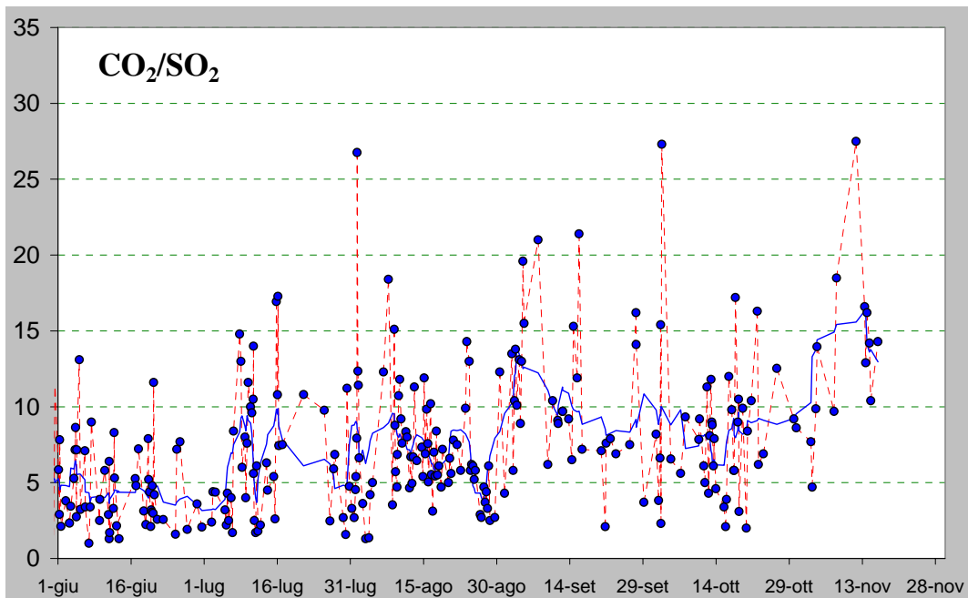
Figura 3– Rapporto \text{CO}_2/\text{SO}_2 misurato nel plume vulcanico dello Stromboli nel periodo tra il 1 giugno e il 18 novembre 2014 (ultimo dato ore 7:30 locali del 16 novembre).
