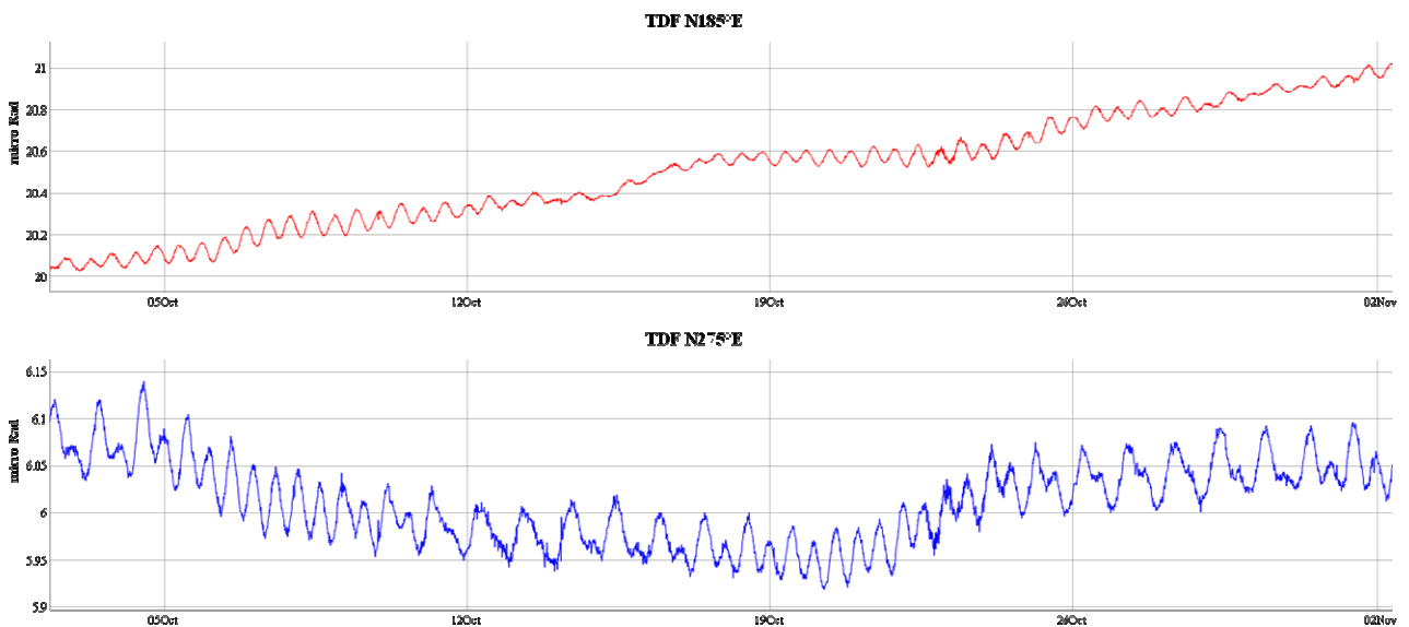
Figura 8 - Dato clinometrico nel periodo compreso tra il 2 ottobre ed il 2 novembre 2014.
