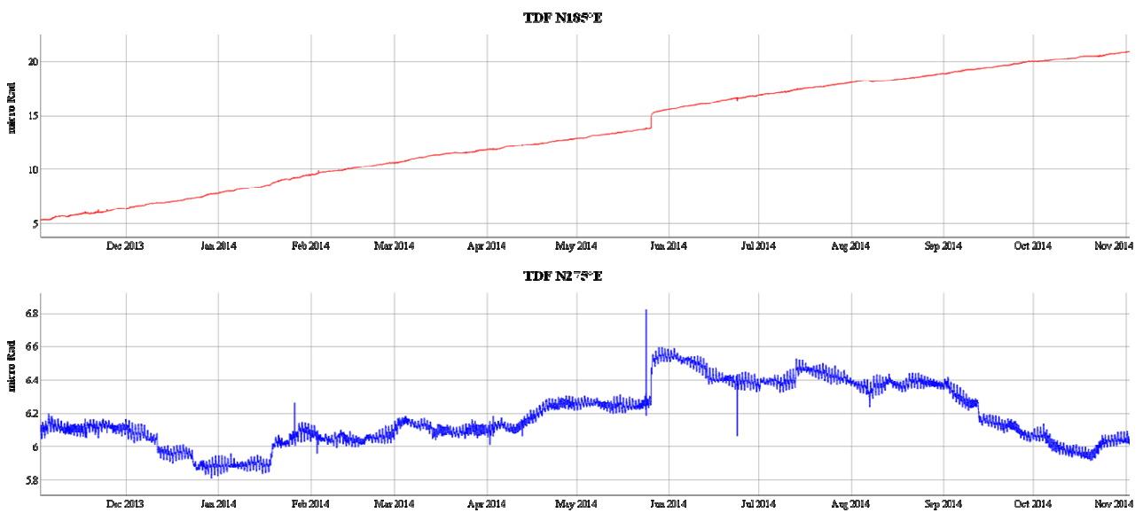
Figura 7 - Dato clinometrico nel periodo compreso tra novembre 2013 ed novembre 2014.
