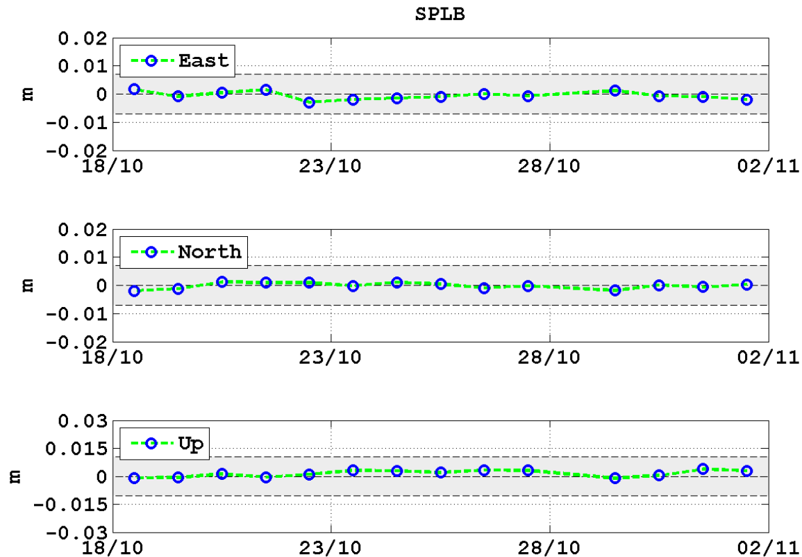
Figura 9 - Serie temporali delle componenti E-W, N-S e quota per gli ultimi 15 giorni delle stazioni CGPS dello Stromboli, calcolate attraverso il software RTD.
