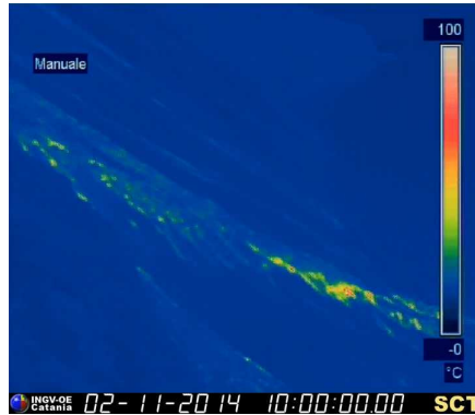
Figura 2 – Immagine termica ripresa dalla telecamera di quota 190 m che mostra accumulo di blocchi caldi alla base della Sciara del Fuoco.
