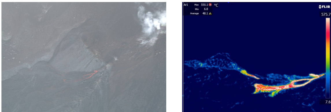
Figura 3 – Immagine visibile (a sinistra) e termica (a destra) del campo lavico attivo ripresa durante il sorvolo con l’elicottero della Guardia Costiera.
