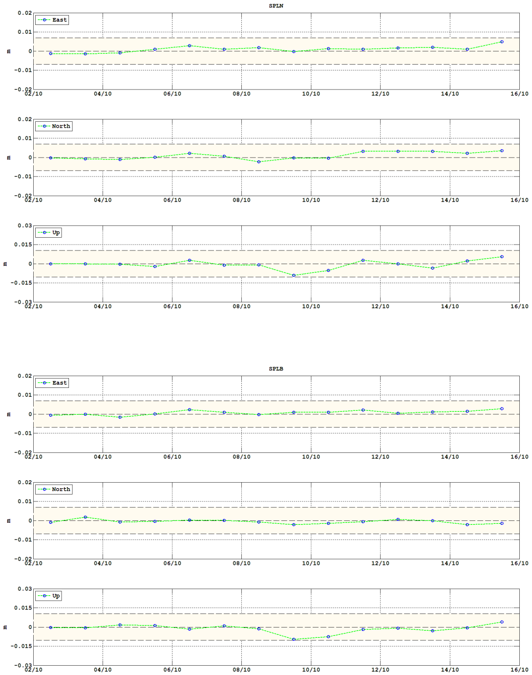
Figura 9 - Serie temporali delle componenti E-W, N-S e quota per gli ultimi 15 giorni delle stazioni CGPS dello Stromboli, calcolate attraverso il software RTD.
