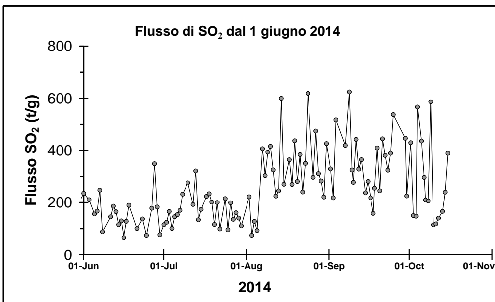
Figura 6 – Flusso di SO 2 medio-giornaliero dal 1 giugno del 2014.
