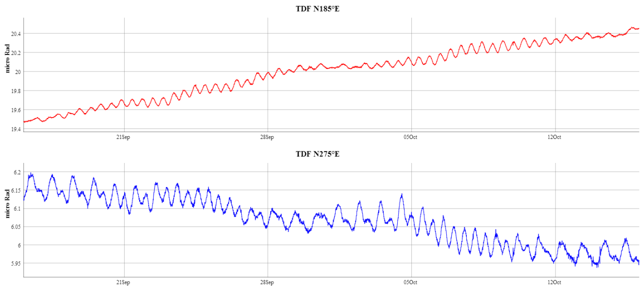
Figura 8 - Dato clinometrico nel periodo compreso tra il 14 settembre ed il 16 ottobre 2014.
