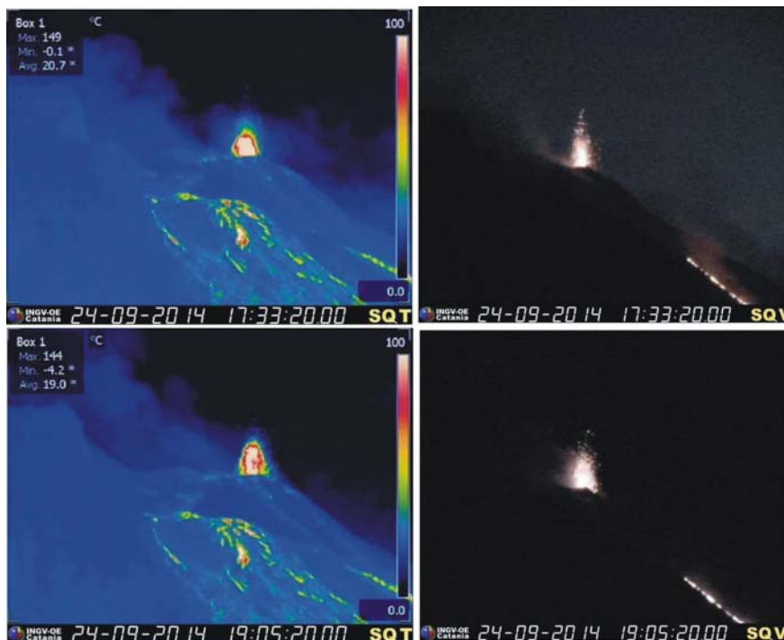
Figura 1 – Immagini riprese dalle telecamere termica e visibile di quota 400 m che mostrano le esplosioni caratterizzate dal lancio di brandelli lavici avvenute nel settore meridionale dell'area craterica.
