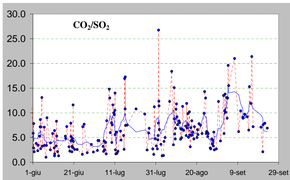
Figura 5 – Rapporto \text{CO}_2/\text{SO}_2 misurato nel plume vulcanico dello Stromboli nel periodo tra il 1 giugno e il 23 settembre 2014 (ultimo dato ore 11:30 locali del 23 settembre).
