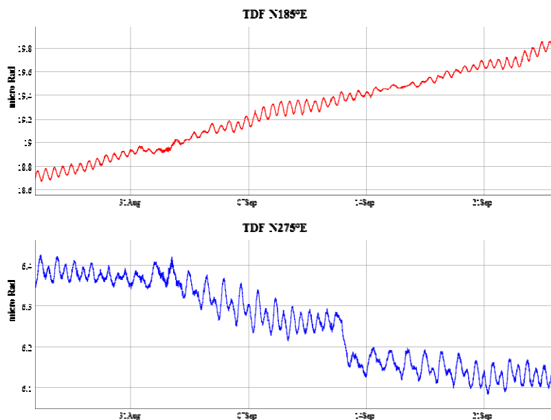
Figura 11 - Dato clinometrico nel periodo compreso tra il 20 agosto e il 24 settembre 2014.
