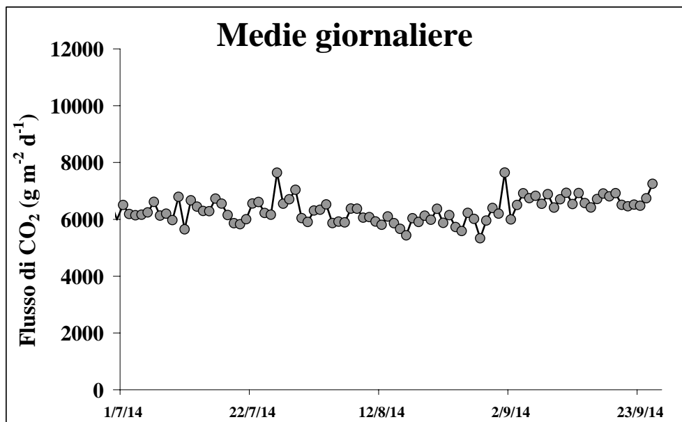
Figura 4 - Flusso medio-giornaliero di \text{CO}_2 dal suolo nel periodo tra il 1 luglio ed il 25 settembre 2014.
