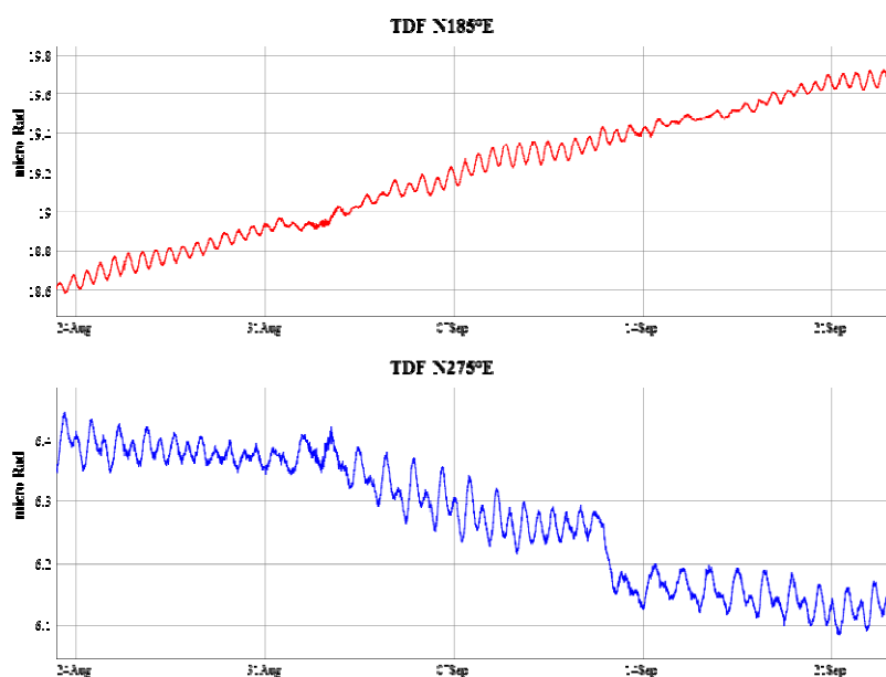
Figura 11 - Dato clinometrico nel periodo compreso tra il 20 agosto e il 22 settembre 2014.
