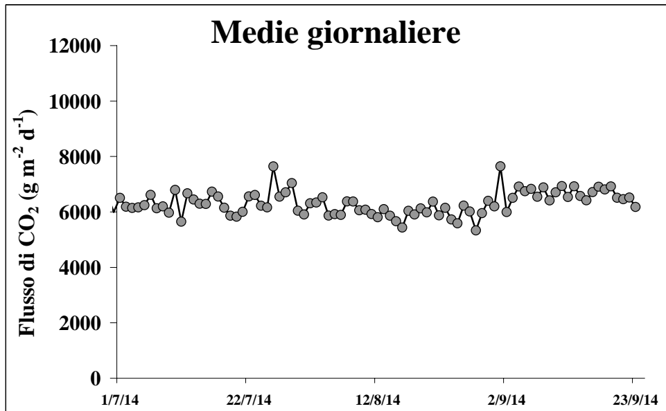
Figura 4 - Flusso medio-giornaliero di CO_2 dal suolo nel periodo tra il 1 luglio ed il 23 settembre 2014.
