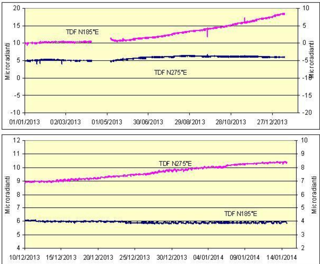
Fig. 3.1 Variazione dell'inclinazione del suolo alla stazione clinometrica di TDF. Sono riportate le componenti N185°E e N275°le di TDF nel lungo e nel breve periodo.
