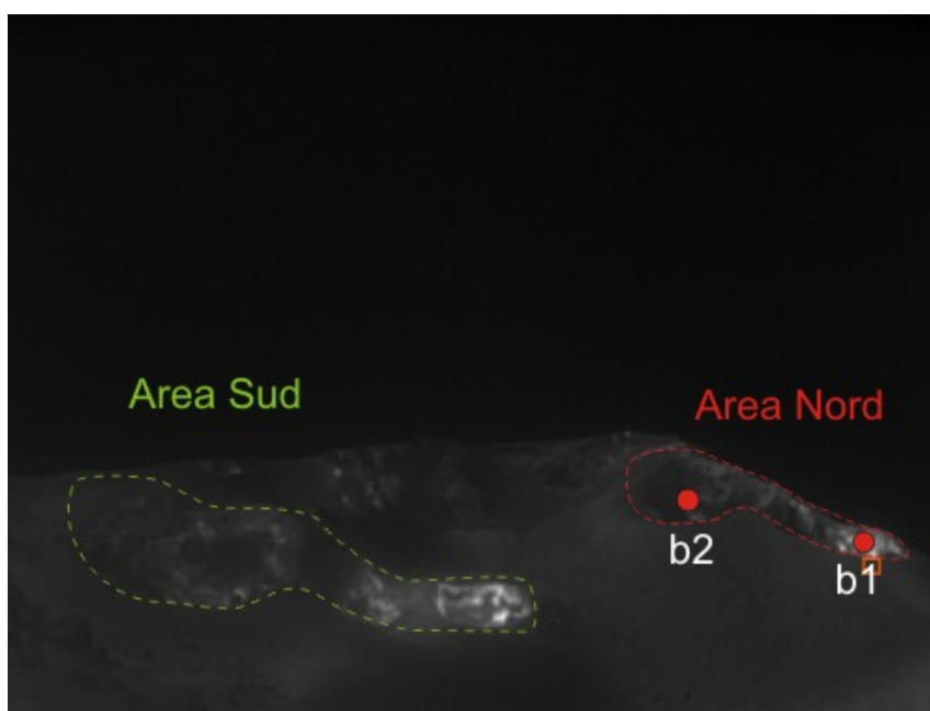
Fig. 1.1 La terrazza craterica vista dalla telecamera del sistema CERBERUS il giorno 03 agosto, con la delimitazione delle aree sedi di bocche attive e l'ubicazione delle due bocche attive nell'Area Nord.
