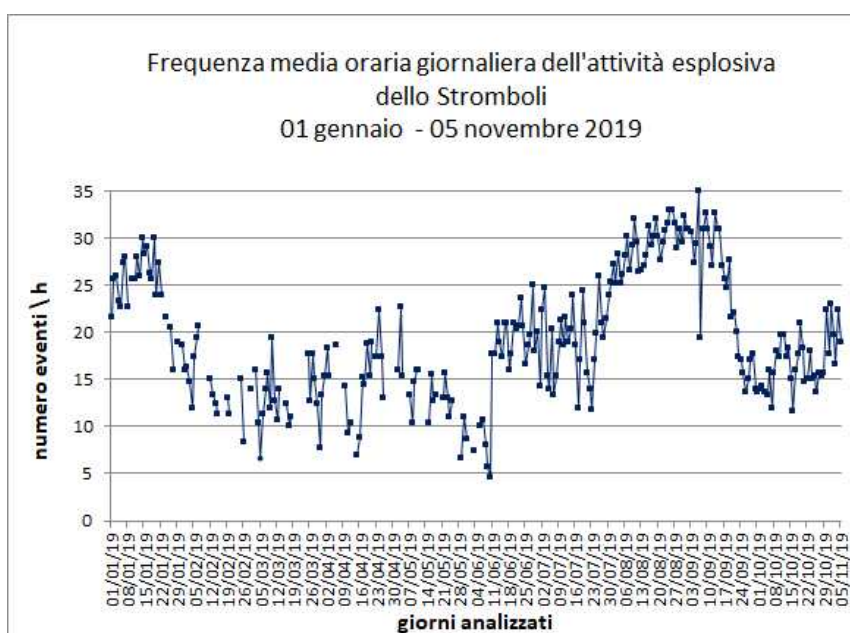
Fig. 3.2 - Frequenza media oraria giornaliera totale delle esplosioni dello Stromboli tra gennaio e novembre 2019 (dato aggiornato al 5 novembre)
