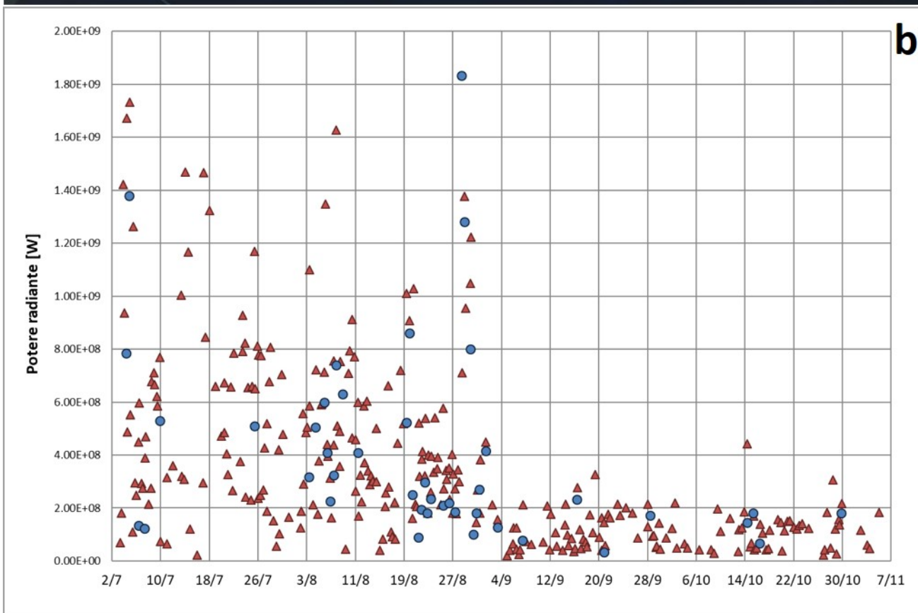
Fig. 7.1 - a) RGB composita delle bande 7, 5 e 4 dell'immagine Landsat 8 del 3 novembre 2019, 09h:41m GMT (risoluzione spaziale 30m), in cui è visibile l'anomalia termica associata all'attività sommitale. b) Flusso radiante calcolato da dati MODIS (triangolo rosso) e Sentinel-3 SLSTR (cerchio blu) dal 3 luglio al 5 novembre.
