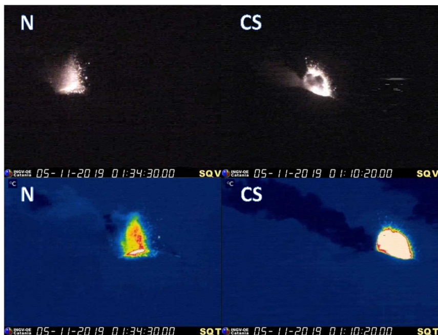
Fig. 3.1 - Immagini sul visibile e sul termico riprese dalla rete di monitoraggio telecamere posta a quota 400 m che mostra l'attività esplosiva prodotta dall'area Nord (N) e da quella Centro Sud (CS).
