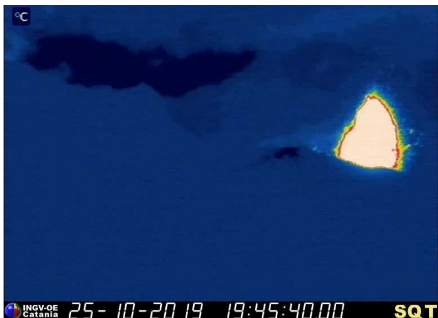
Fig. 3.2 - Immagine termica di un'esplosione dell'area S, le riprese sono da quota 400 m (s.l.m).
