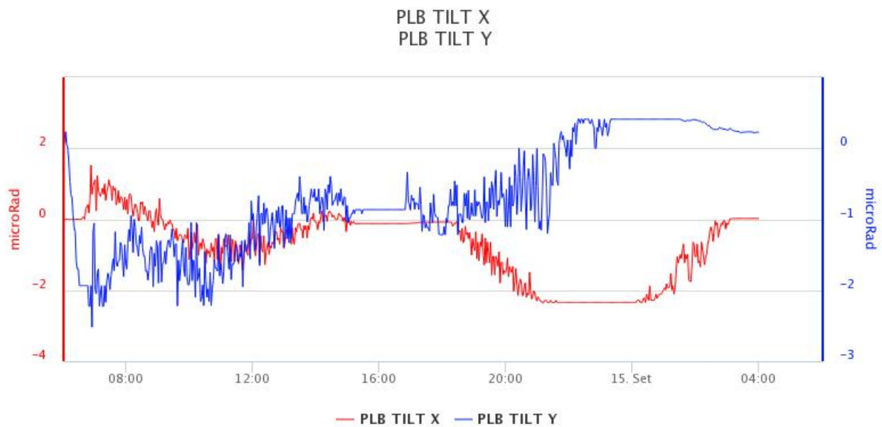
Fig. 5.2 - Componenti X e Y del tilt di PLB
