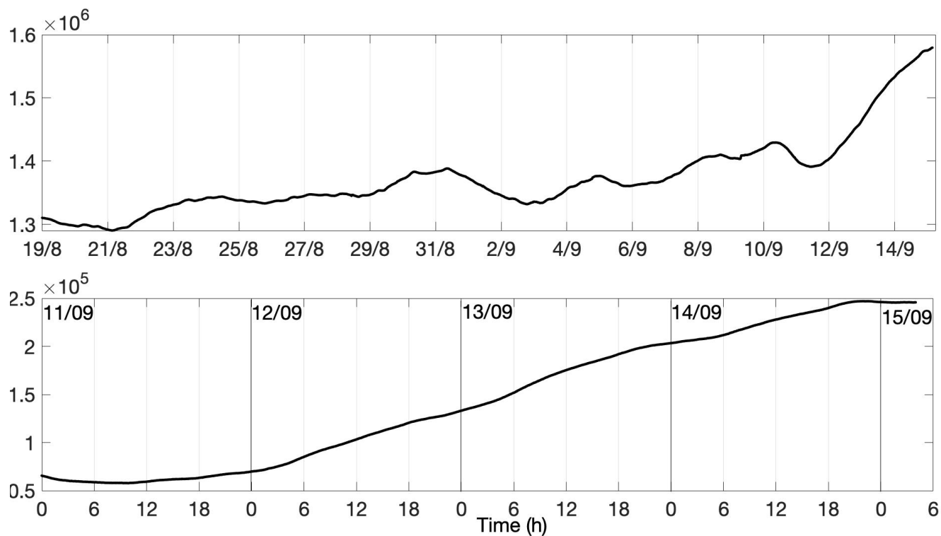
Fig. 4.3 - Grafico relativo al dato dilatometrico registrato a SVO: in alto viene mostrato lo strain registrato dal 19 agosto, in basso dall' 11 settembre al 15 settembre, ore 5:00 UTC.
