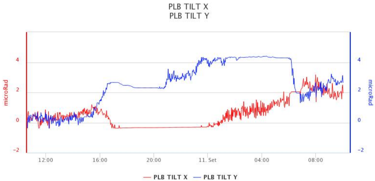
Fig. 5.2 - Componenti X e Y della stazione PLB
