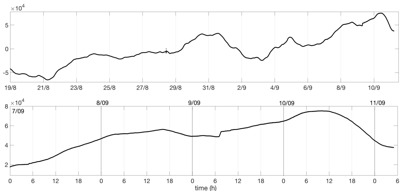
Fig. 4.3 - Grafico relativo al dato dilatometrico registrato a SVO: in alto viene mostrato lo strain registrato dal 19 agosto, in basso dal 7 settembre al 11 settembre, ore 5:00 UTC.
