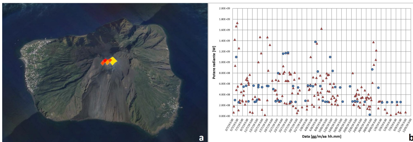
Fig. 7.1 - a) Anomalie termiche associate all'attività sommitale ricavata dall'immagine ASTER (banda 13) dell'8 settembre 2019, 21h:03m GMT. b) Flusso radiante calcolato da dati MODIS (triangolo rosso) e Sentinel-3 SLSTR (cerchio blu) dal 3 luglio al 10 settembre.
