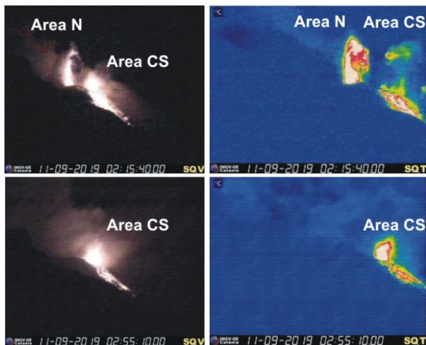
Fig. 3.1 - Attività stromboliana da due delle bocche attive all'interno delle due aree crateriche N e CS.
