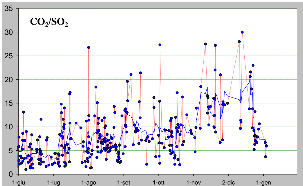
Figura 2– Rapporto \text{CO}_2/\text{SO}_2 misurato nel plume vulcanico dello Stromboli nel periodo tra il 1 giugno e il 4 gennaio 2015 (ultimo dato ore 6:30 locali del 4 gennaio).
