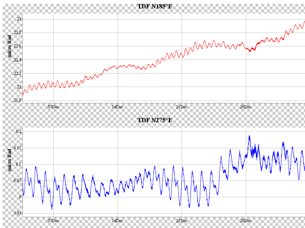
Fig.8 - Dato clinometrico nel periodo compreso tra il 30 novembre 2014 e il 03 gennaio 2015
