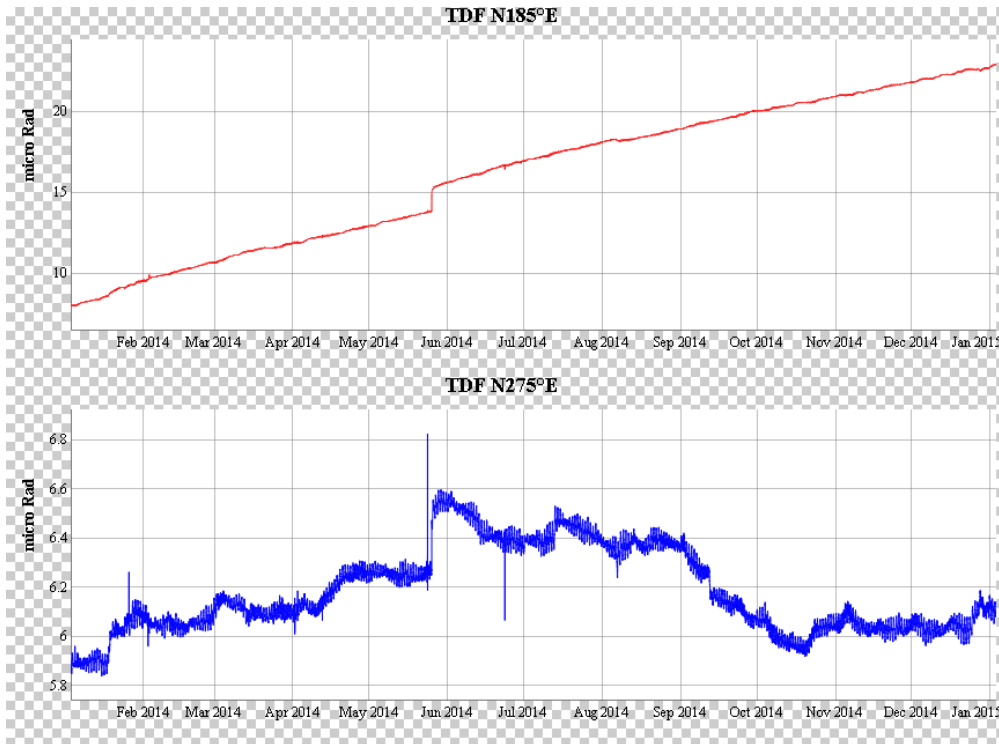
Fig.7- Dati clinometrici nel periodo compreso tra gennaio 2014 e gennaio 2015
