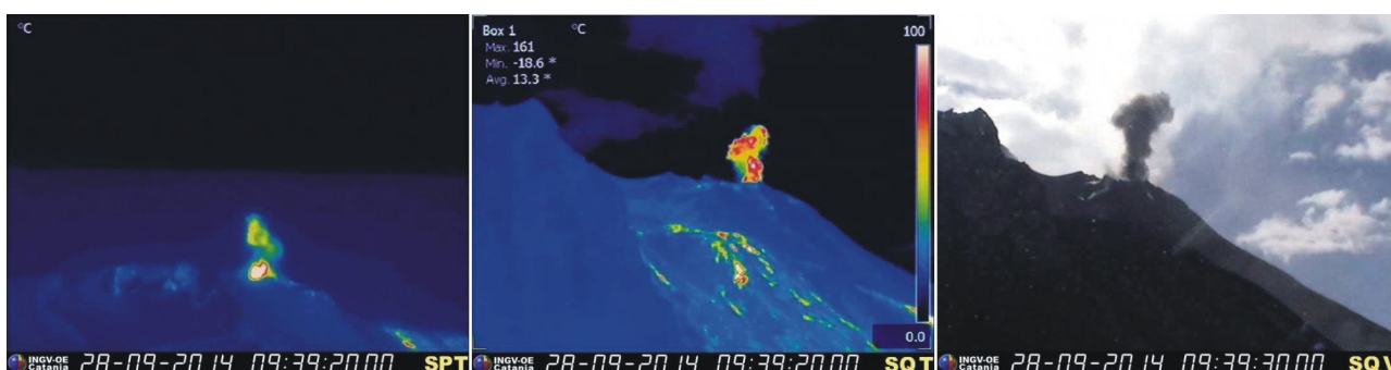
Figura 1 – Immagini riprese dalla telecamere termica del Pizzo e dalle telecamere visibile e termica di quota 400 m che mostrano un emissione di cenere avvenuta dal settore meridionale dell'area craterica. L'immagine termica al centro di quota 400 m mostra, inoltre, la colata attiva che è visibile in basso a destra in corrispondenza del fondo scala dell'immagine.
