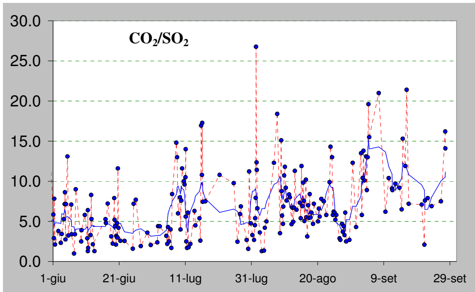
Figura 4 – Rapporto CO_2/SO_2 misurato nel plume vulcanico dello Stromboli nel periodo tra il 1 giugno e il 27 settembre 2014 (ultimo dato ore 17:30 locali del 27 settembre).
