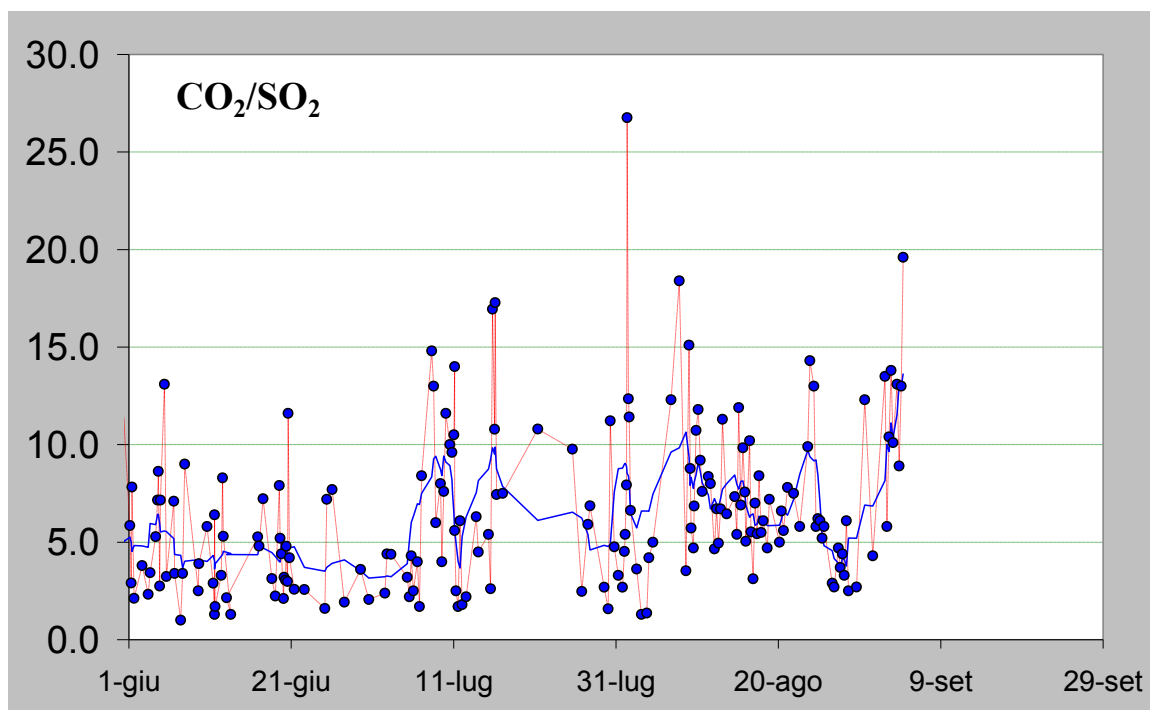
Figura 4 – Rapporto CO 2 /SO 2 misurato nel plume vulcanico dello Stromboli nel periodo tra il 1 giugno ed il 4 settembre 2014 (ultimo dato ore 11:30 locali del 4 settembre).
