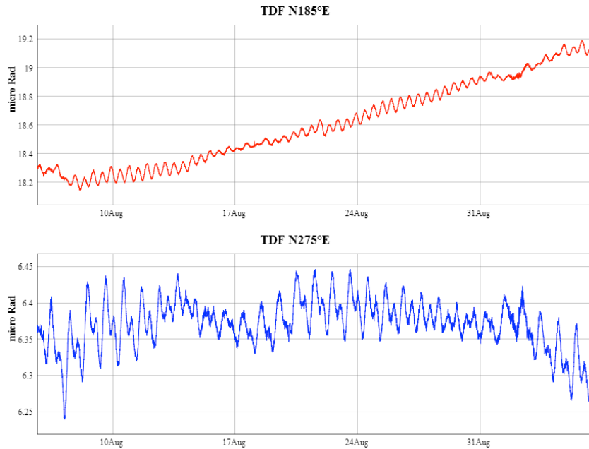
Figura 10 – Dato clinometrico nel periodo compreso tra inizio agosto e il 5 settembre 2014
