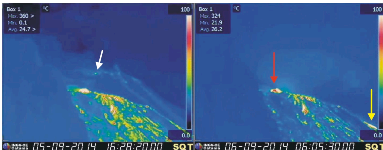
Figura 1 - Immagini termiche della telecamera di quota 400 m s.l.m. Nell'immagine a sinistra la freccia bianca indica una piccola anomalia termica che interessa la terrazza craterica, probabilmente causata da un'attività di degassamento impulsivo. Nell'immagine a destra la freccia rossa indica approssimativamente la posizione della bocca effusiva di quota 650 m che genera la colata lavica. Rispetto a ieri, la quantità di lava che tracima dal pianoro di quota 600 m appare in generale diminuzione, soprattutto nella porzione settentrionale del campo lavico. Dalle ore 05.00 UTC circa di oggi si nota un'anomalia termica posizionata nella parte meridionale del campo lavico (indicata con la freccia gialla) che potrebbe essere generata ad una nuova piccola tracimazione lavica.
