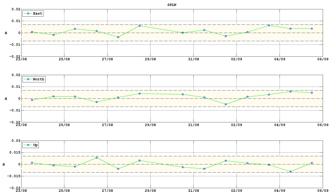
Figura 8 – Dati GPS della stazione di Punta Lena del periodo 23/8/2014 – 5/9/2014.
