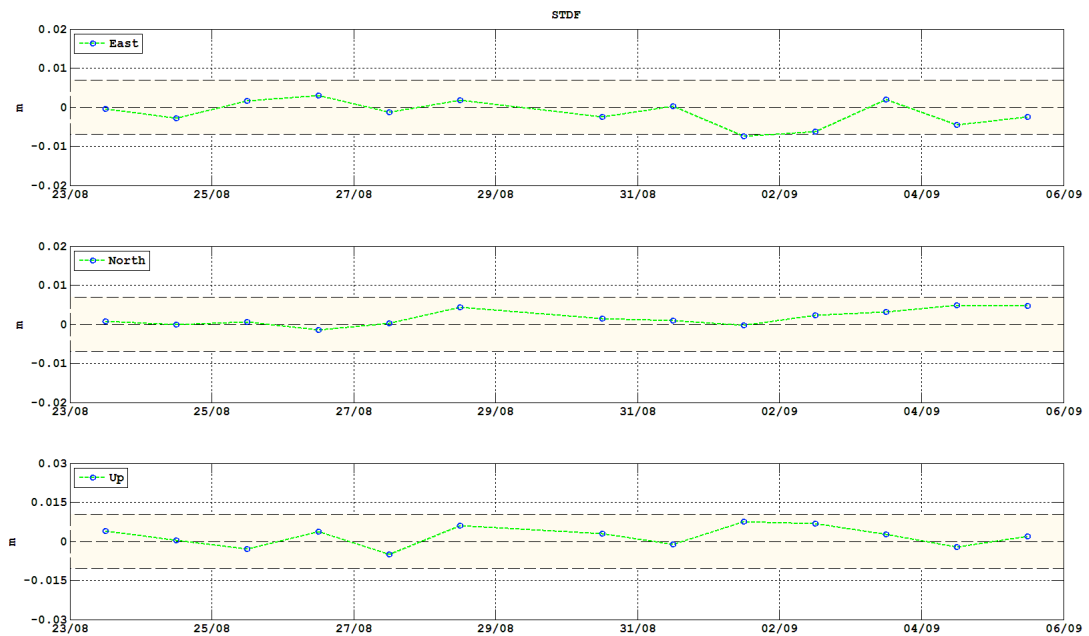
Figura 7 – Dati CGPS della stazione di Timpone del Fuoco del periodo 23/8/2014 – 5/9/2014.
