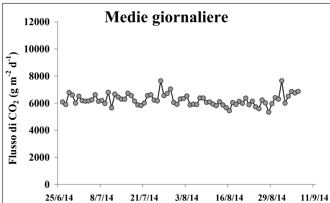
Figura 3 – Flusso medio-giornaliero di CO 2 dal suolo nel periodo tra il 25 giugno ed il 6 settembre 2014
