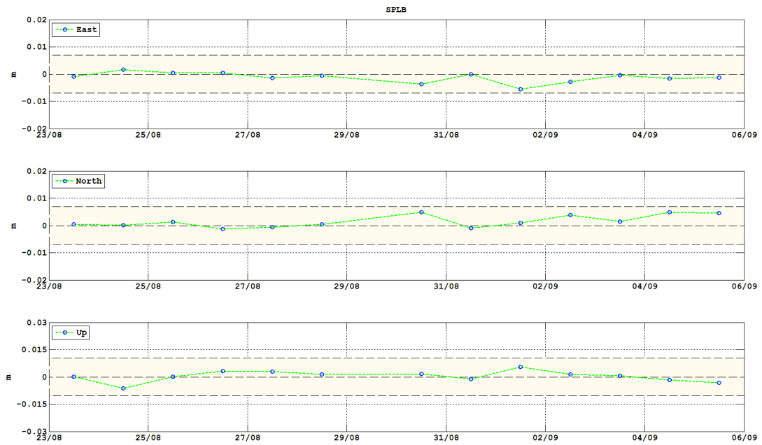
Figura 6 – Dati GPS della stazione di Punta Labronzo del periodo 23/8/2014 – 5/9/2014.
