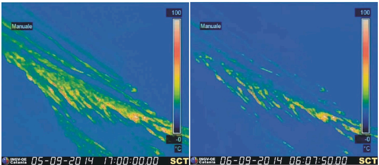
Figura 2 – Nelle immagini termiche della telecamera di quota 190 è visibile la parte più bassa del campo lavico, che si presenta in raffreddamento. La zona è interessata unicamente dal rotolio di blocchi lavici provenienti in prevalenza dalle zone dei fronti lavici attivi più a monte.
