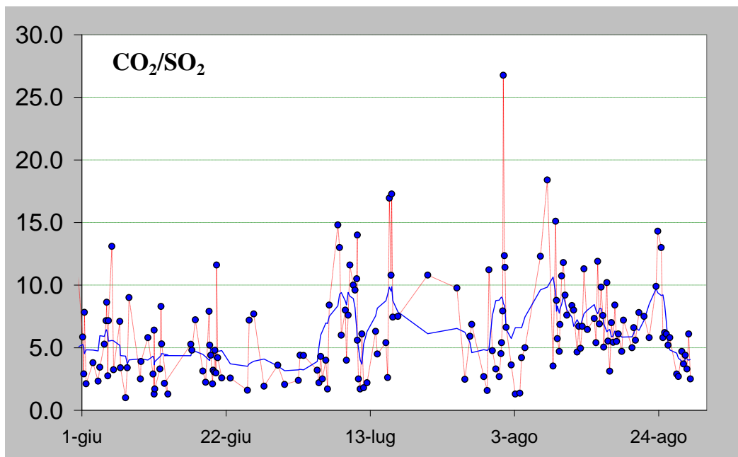
Figura 4 – Rapporto CO_2/SO_2 misurato nel plume vulcanico dello Stromboli nel periodo tra il 1 giugno ed il 29 agosto 2014 (ultimo dato ore 17:30 locali del 28 agosto).
