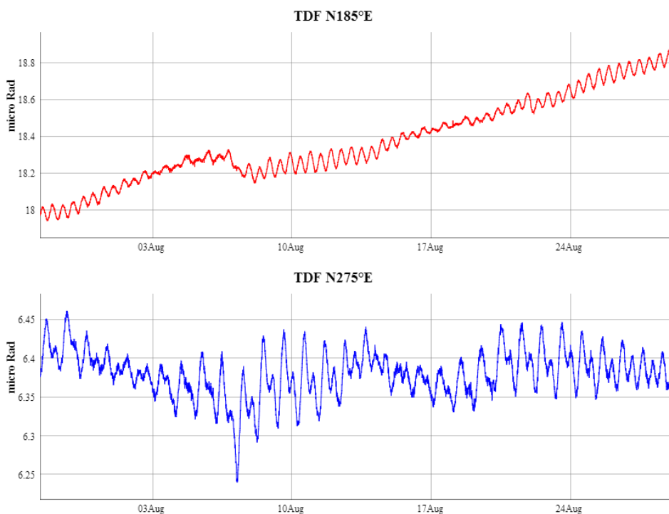
Figura 10 – Dato clinometrico nel periodo compreso tra luglio e il 28 agosto 2014
