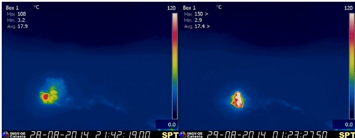
Figura 1 – Immagini termiche della telecamera del Pizzo, acquisite alle ore 21:42 UTC del 28 agosto e alle ore 01:23 UTC del 29 agosto, relative all'area craterica sommitale. Si osservano chiare anomalie termiche, anche particolarmente forti come nel caso dell'immagine di destra, che segnalano eventi di degassamento impulsivo ad alta temperatura dovuti ad attività esplosiva nell'area craterica Sud. In basso a destra in entrambe l'immagini si osserva l'anomalia termica corrispondente alla bocca effusiva che alimenta le colate laviche lungo la Sciara del Fuoco.
