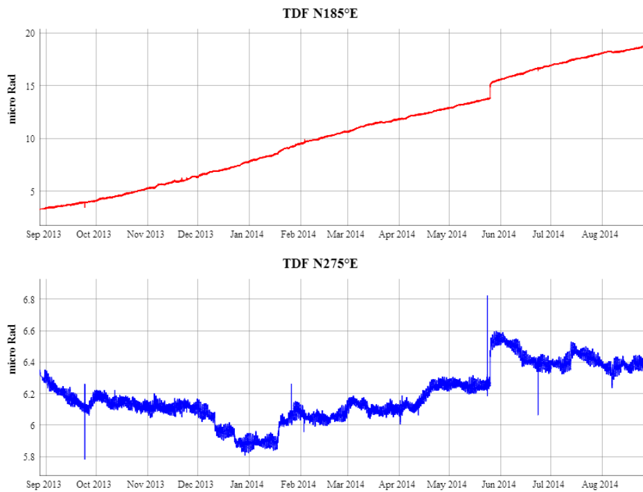
Figura 9– Dato clinometrico nel periodo compreso tra Settembre 2013 e agosto 2014
