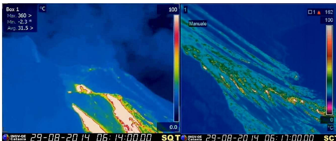
Figura 2 – Immagini termiche delle telecamere di quota 400 m s.l.m. a sinistra e 190 m s.l.m. a destra acquisite, rispettivamente, alle ore 06:14 e 06:17 UTC di oggi.
