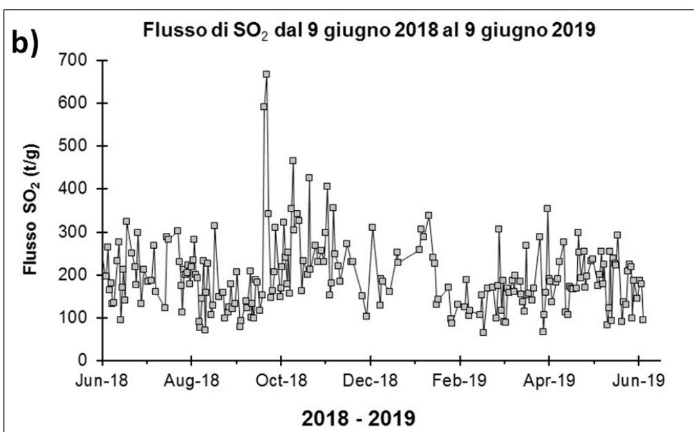
Fig. 6.1 - Andamento temporale del flusso di SO 2 nel corso dell'ultimo mese (a) e dell'ultimo anno (b)
