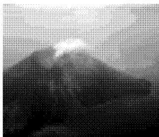
Il vulcano di Stromboli
