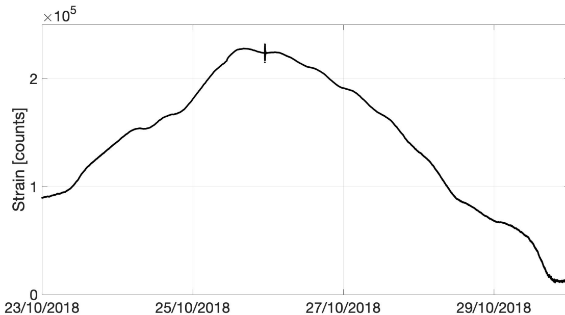
Fig. 4.4 - Grafico relativo ai dati dilatometrici registrati a SVO: in nero viene mostrato il dato processato, ripulito dalle maree.
