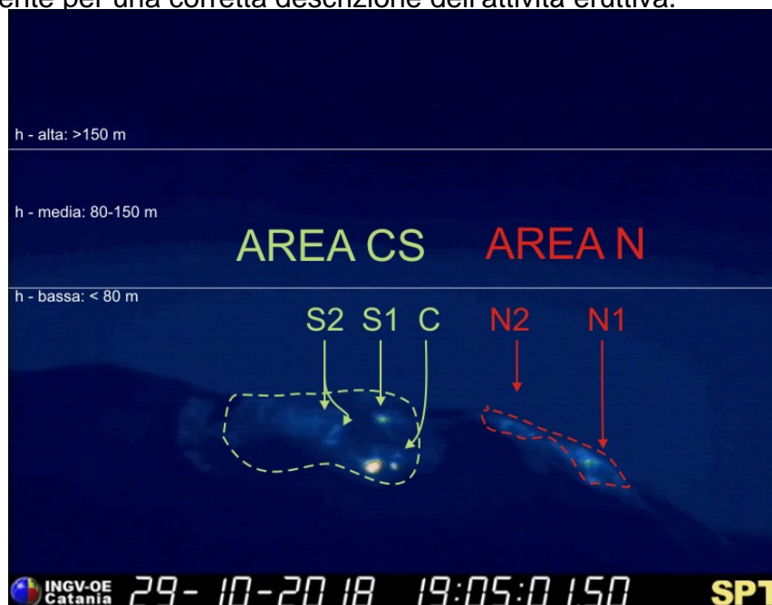
Fig. 3.1 - La terrazza craterica vista dalla telecamera termica posta sul Pizzo sopra la Fossa con i settori in cui è divisa (AREA N, AREA C-S). Le sigle e le frecce indicano i nomi e le ubicazioni delle bocche attive. L'areale soprastante la terrazza craterica è diviso in tre intervalli di altezze ( h ) che indicano l'intensità dell'esplosioni.
