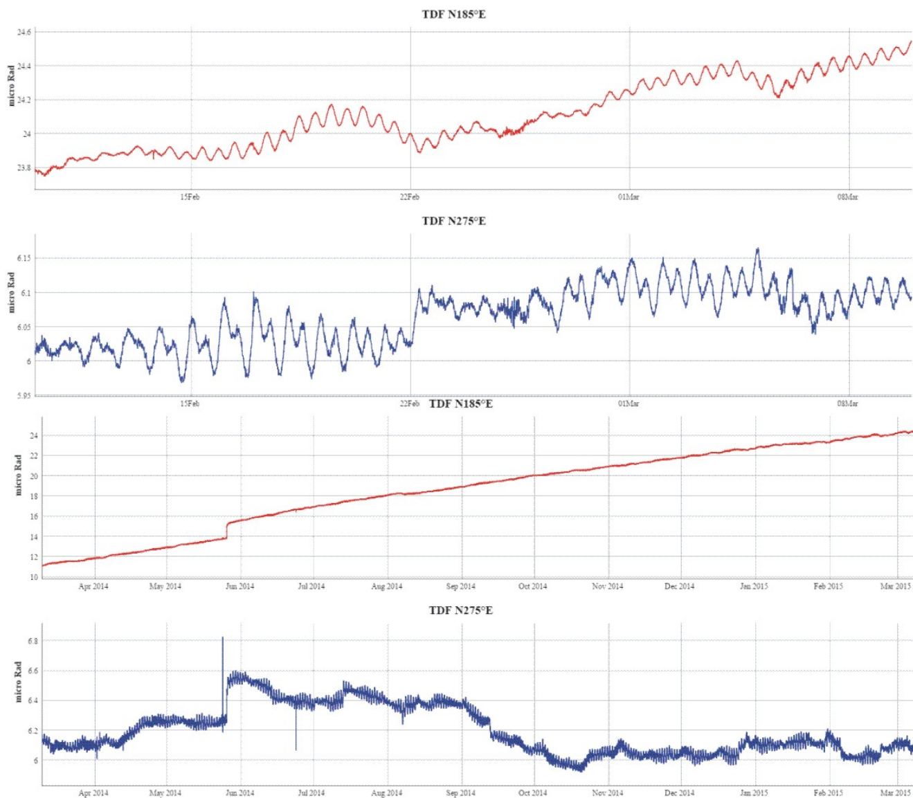
Fig. 3.1 Variazione dell'inclinazione del suolo alla stazione clinometrica di TDF. Sono riportate le componenti N185°E e N275°le di TDF nel breve (un mese) e nel lungo (un anno) periodo.
