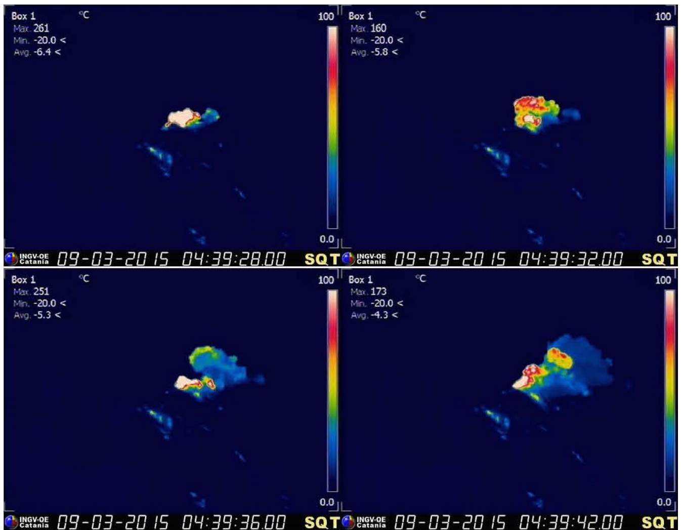
Fig. 1.1 Immagini termiche dell'esplosione stromboliana più intensa registrata in questo periodo, caratterizzata dall'accadimento di due singoli eventi a distanza di circa 10 sec, che è stata prodotta il 9 marzo da una bocca situata nell'area settentrionale della Terrazza Craterica.
