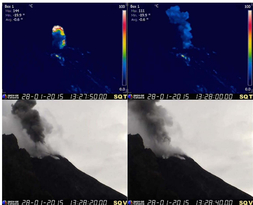
Fig. 1.1 Alcune immagini termiche e in banda visibile dell'esplosione stromboliana più intensa registrata nelle prime ore del 28 gennaio 2015 da una bocca localizzata nell'area craterica settentrionale.
