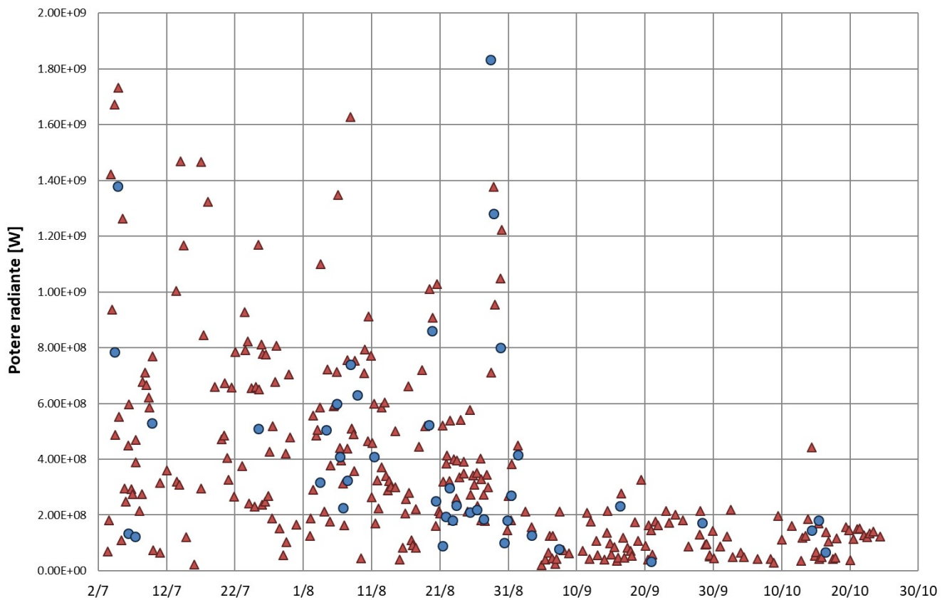
Fig. 7.1 - Flusso radiante calcolato da dati MODIS (triangolo rosso) e Sentinel-3 SLSTR (cerchio blu) dal 3 luglio al 24 ottobre.
