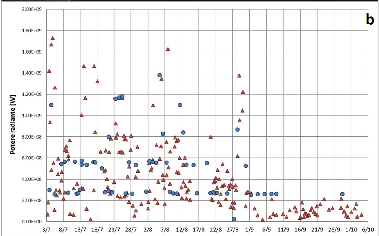
Fig. 7.1 - a) RGB composita dell'immagine Landsat 7 (bande 7, 5 e 4) del 3 ottobre 2019, 09h:20m GMT (risoluzione spaziale 30m). b) Flusso radiante calcolato da dati MODIS (triangolo rosso) e Sentinel-3 SLSTR (cerchio blu) dal 3 luglio al 4 ottobre.
