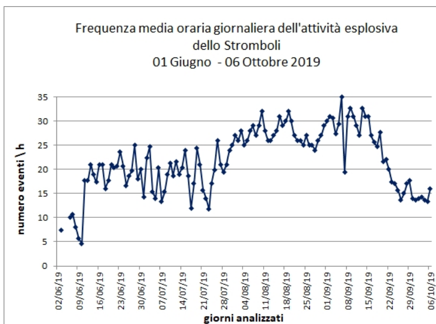
Fig. 3.2 - Frequenza media giornaliera dell'attività esplosiva del vulcano Stromboli, dal 1 giugno al 6 ottobre 2019
