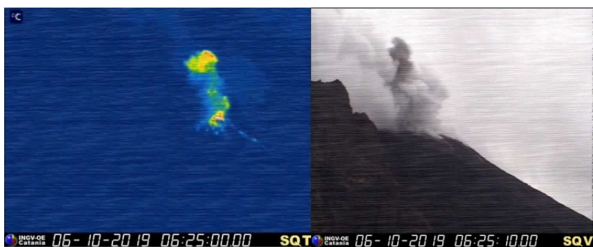
Fig. 3.1 - Immagini estratte dalle telecamere di sorveglianza termica (a sinistra) e visibile (a destra), poste a quota 400 m s.l.m. Si evidenzia l'attività stromboliana che caratterizza le bocche presenti nell'area craterica settentrionale, con emissione di cenere.
