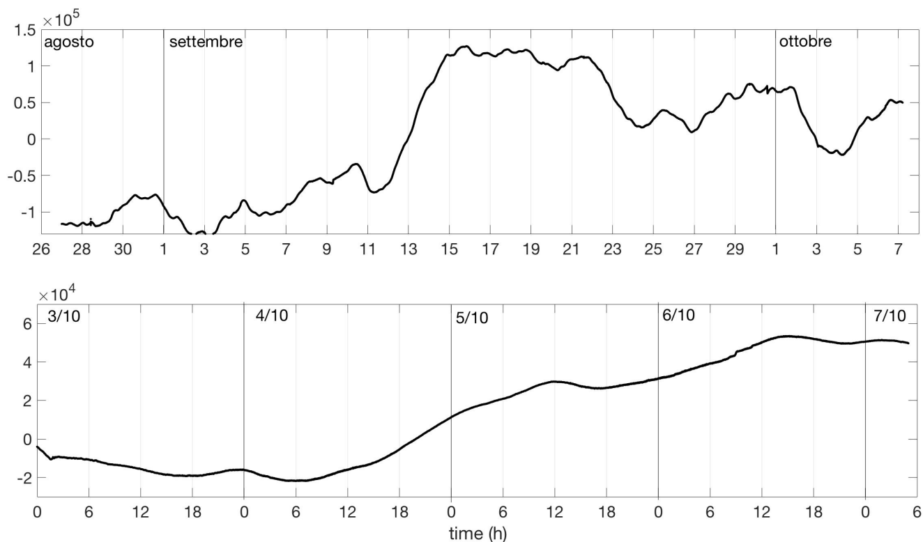
Fig. 4.3 - Grafico relativo al dato dilatometrico registrato alla stazione SVO: in alto viene mostrato lo strain registrato dal 26/08/2019, in basso quello nell'ultima settimana.
