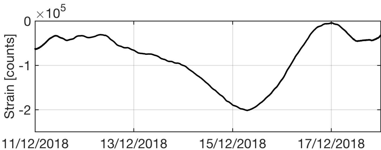
Fig. 4.4 - Grafico relativo ai dati dilatometrici registrati a SVO: viene mostrato il dato processato, ripulito dalle maree.
