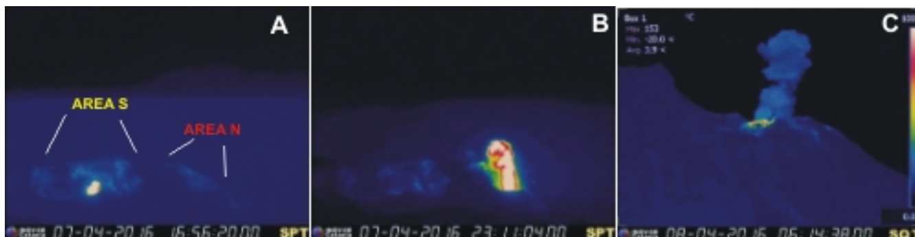
Fig. 1.1 A) e B) - La terrazza craterica ripresa dalla telecamera in banda termica del Pizzo sopra la Fossa. Si osservano le bocche attive nell'area craterica meridionale (A) e in quella settentrionale (B). In (C) si osserva la ricaduta dei prodotti caldi sulla porzione esterna della terrazza craterica durante un'esplosione dell'area craterica settentrionale, ripresa dalla telecamera in banda termica di quota 400.
