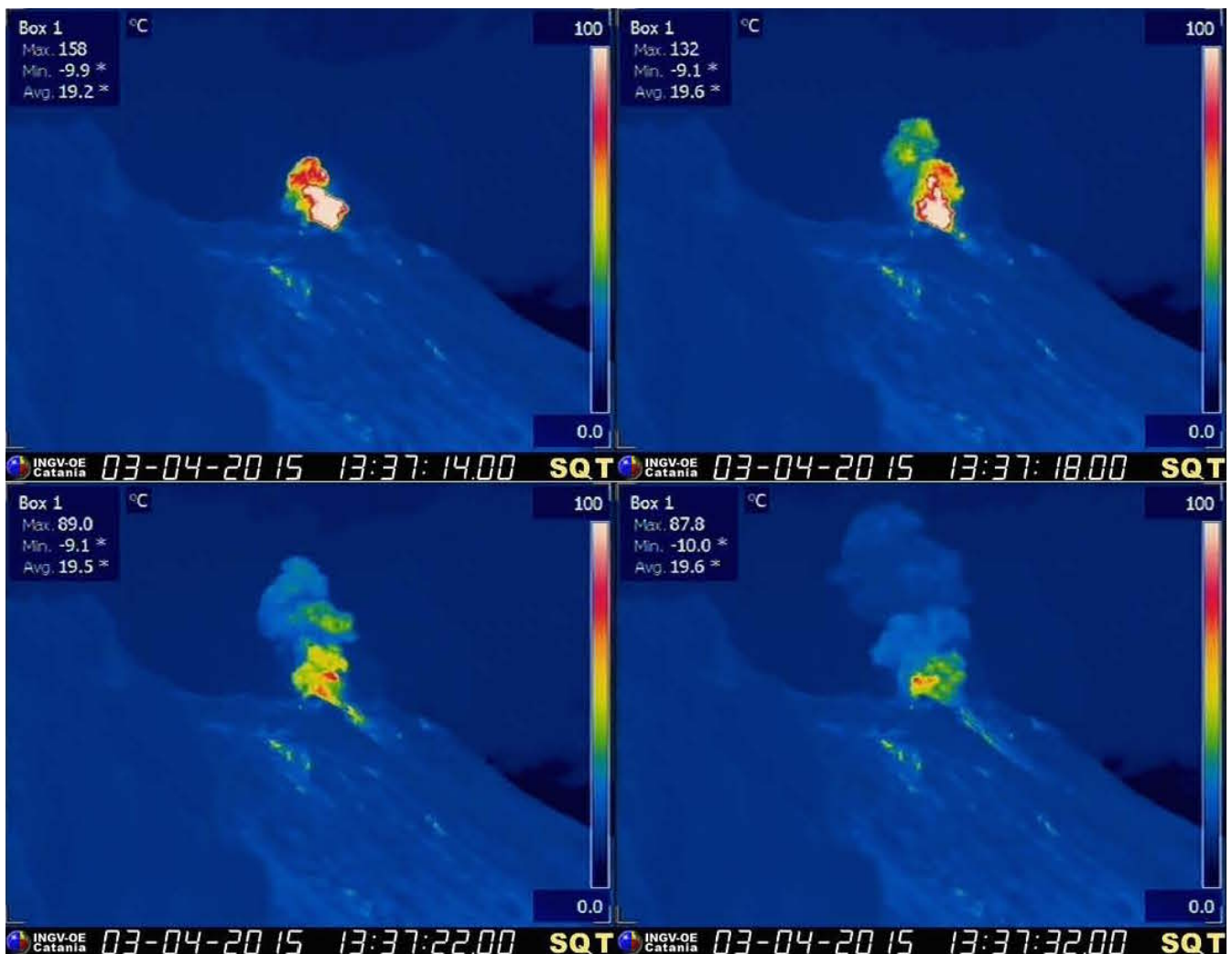
Fig. 1.1 Immagini termiche dell'esplosione stromboliana più intensa del periodo prodotta il 3 aprile da una bocca situata nell'area settentrionale della Terrazza Craterica, e caratterizzata da una serie di pulsazioni susseguitesesi per circa 40 sec.
