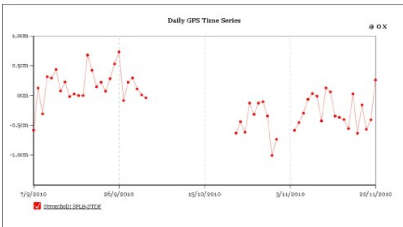
Fig. 3.2 Variazione della Distanza Reale (Slope Distance) tra le stazioni GPS permanenti di Punta Labronzo (SPLB) e Timpone del Fuoco (STDF), nei due intervalli di un anno (in alto) e di due mesi (in basso).
